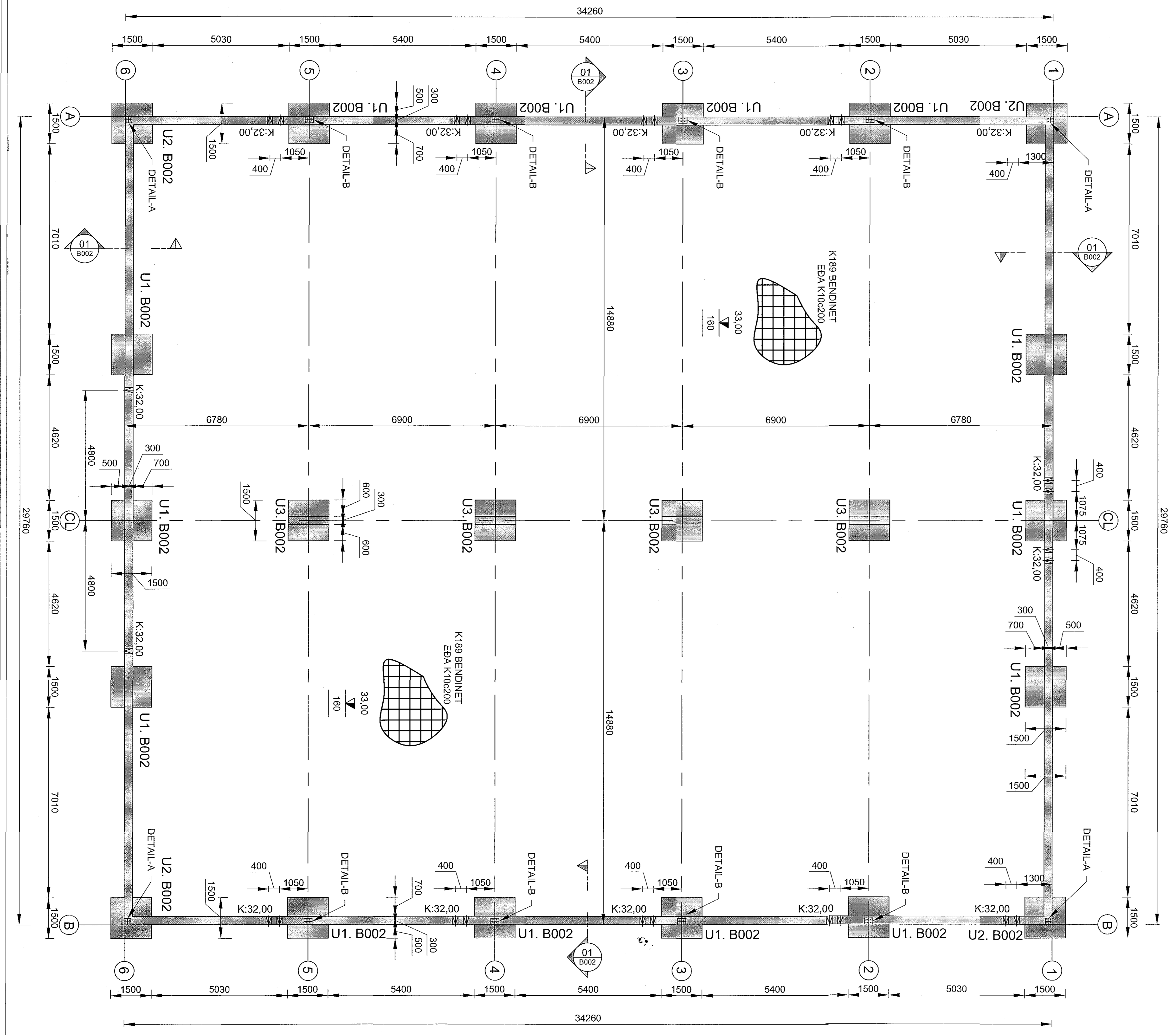
GRUNNMYND - UNDIRSTÖÐUR 1:75 (A1)
