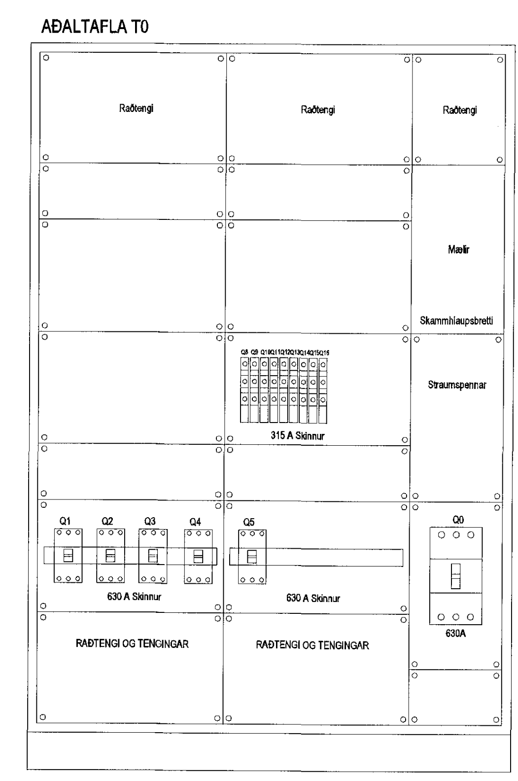
ADALTAFLA T0 TILLAGA AÐ UPPRÖÐUN OG STÆRD BREIDD 105sm HÆÐ 200sm DÝPT 40sm
