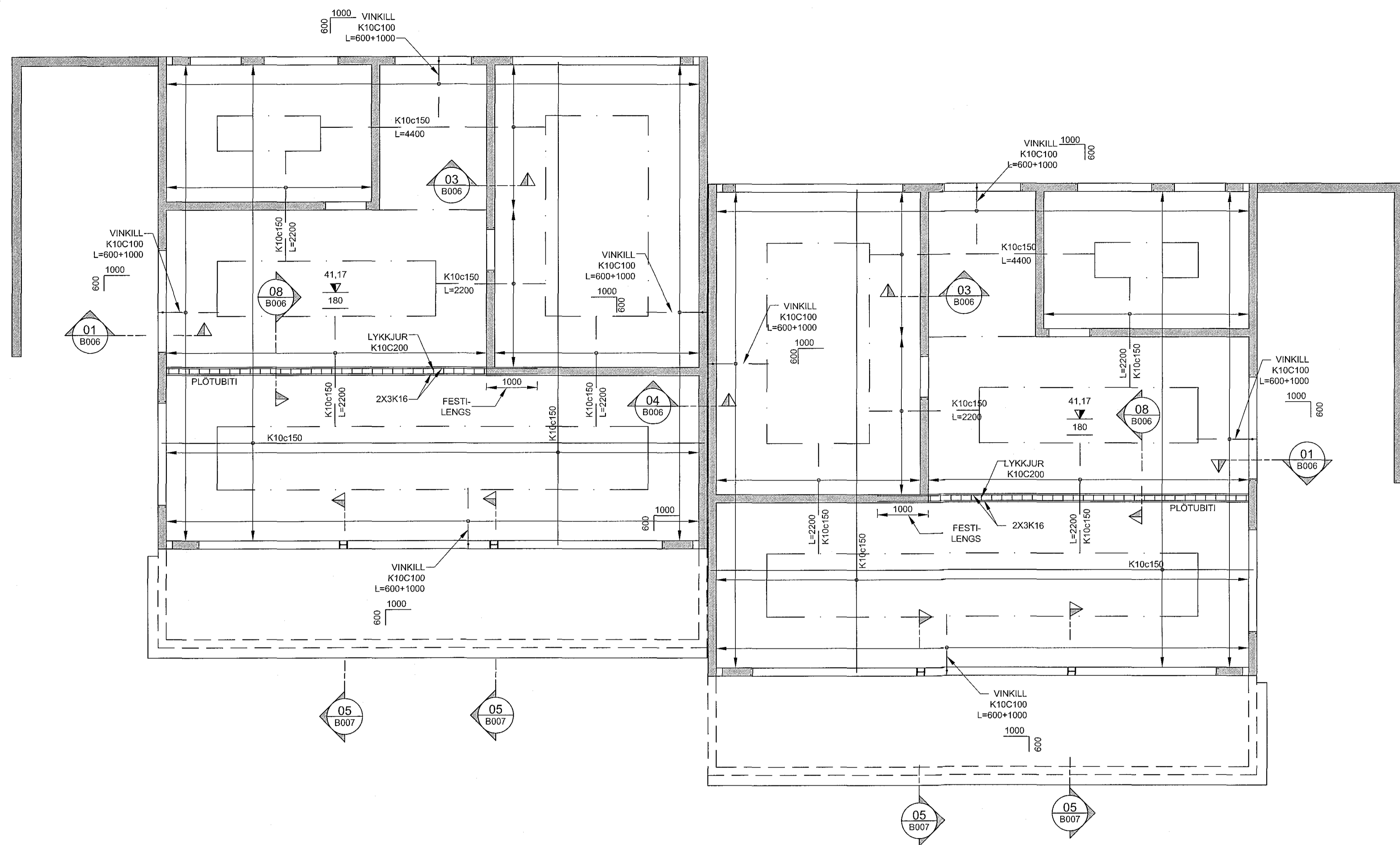
GRUNNMYND - PLATA YFIR 1.HÆÐ. 1:50 (A1)
