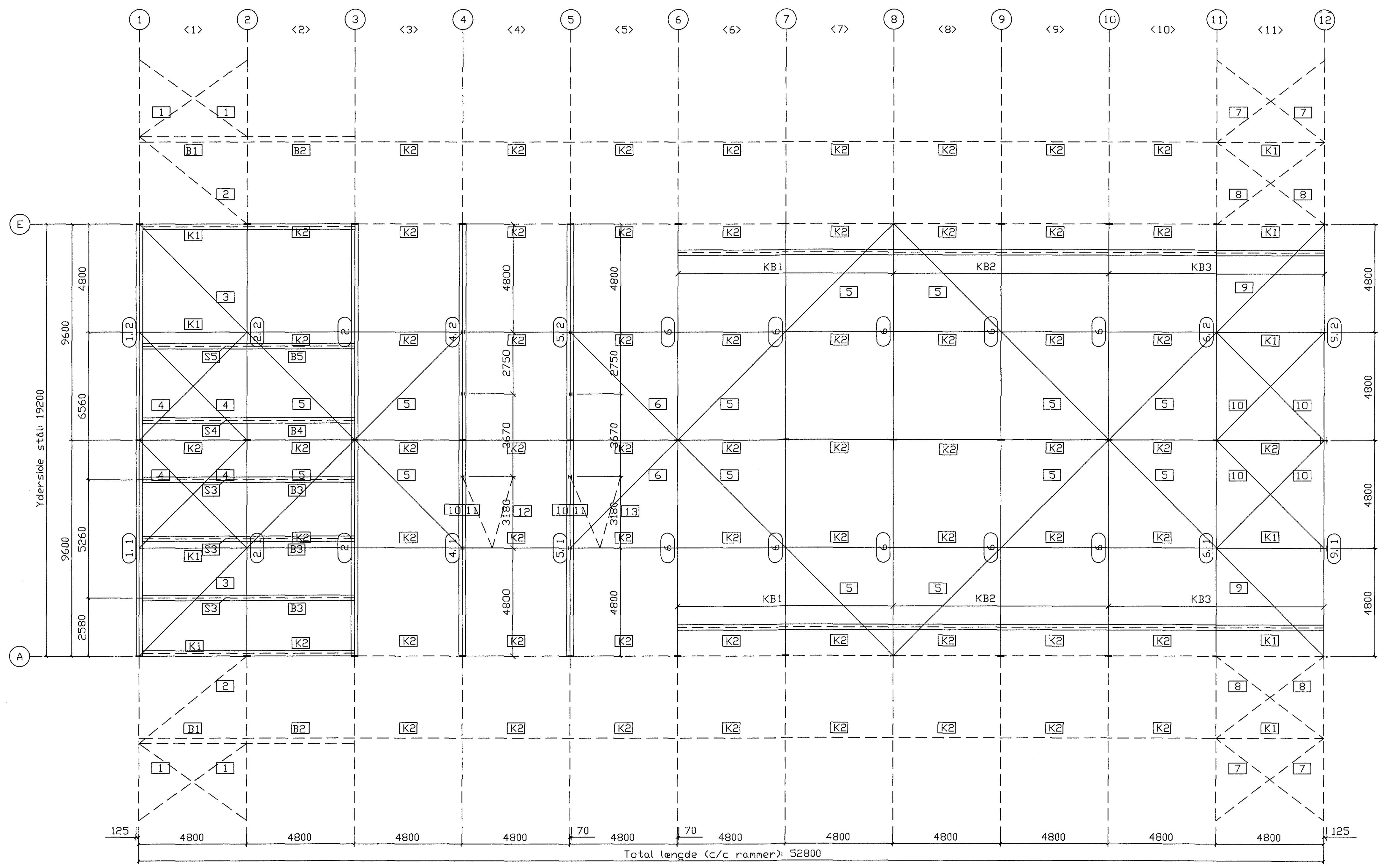
Montageplan Tag og udfoldede facader
