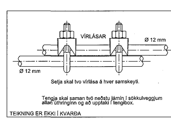
SAMTENGING STEYPUDEINA DEMIGERÐUR FRÁGANÐUR
