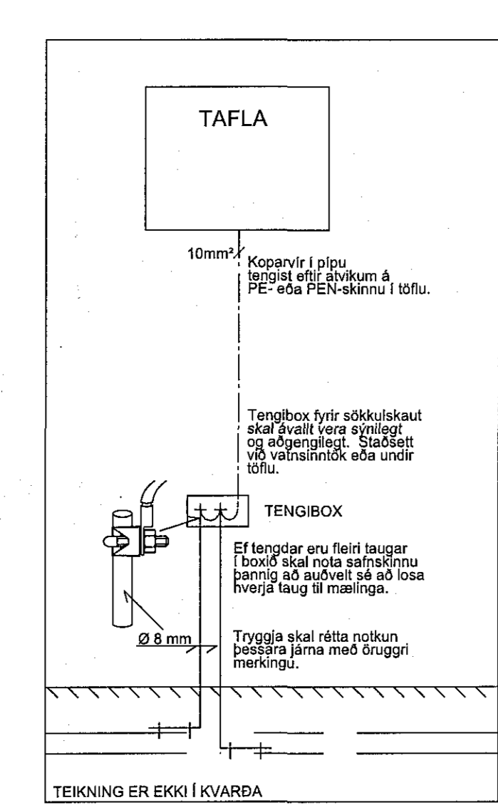
SNID / TOFLUVEGG DEMIGERÐUR FRÁGANÐUR
