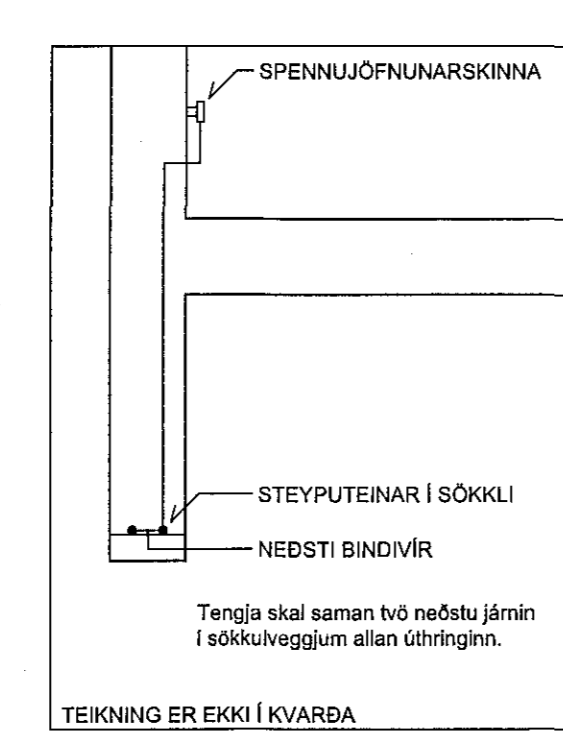
ÞVERSNID / SÖKKLI DEMIGERÐUR FRÁGANÐUR
