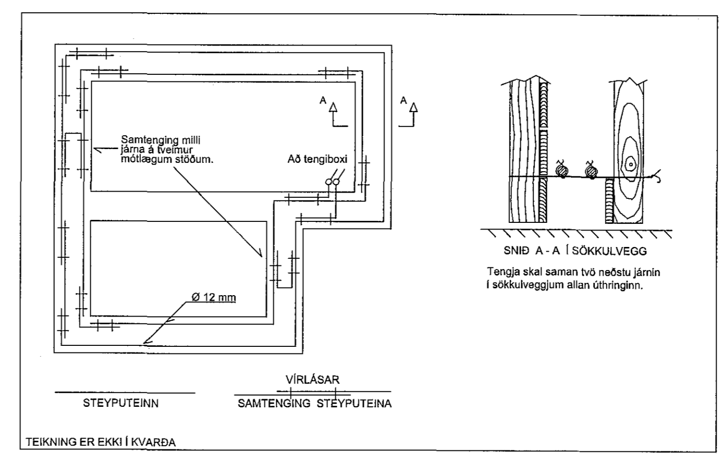
FYRIRMYND GRUNNMYND SÖKKULVEGGJA DEMIGERÐUR FRÁGANÐUR
