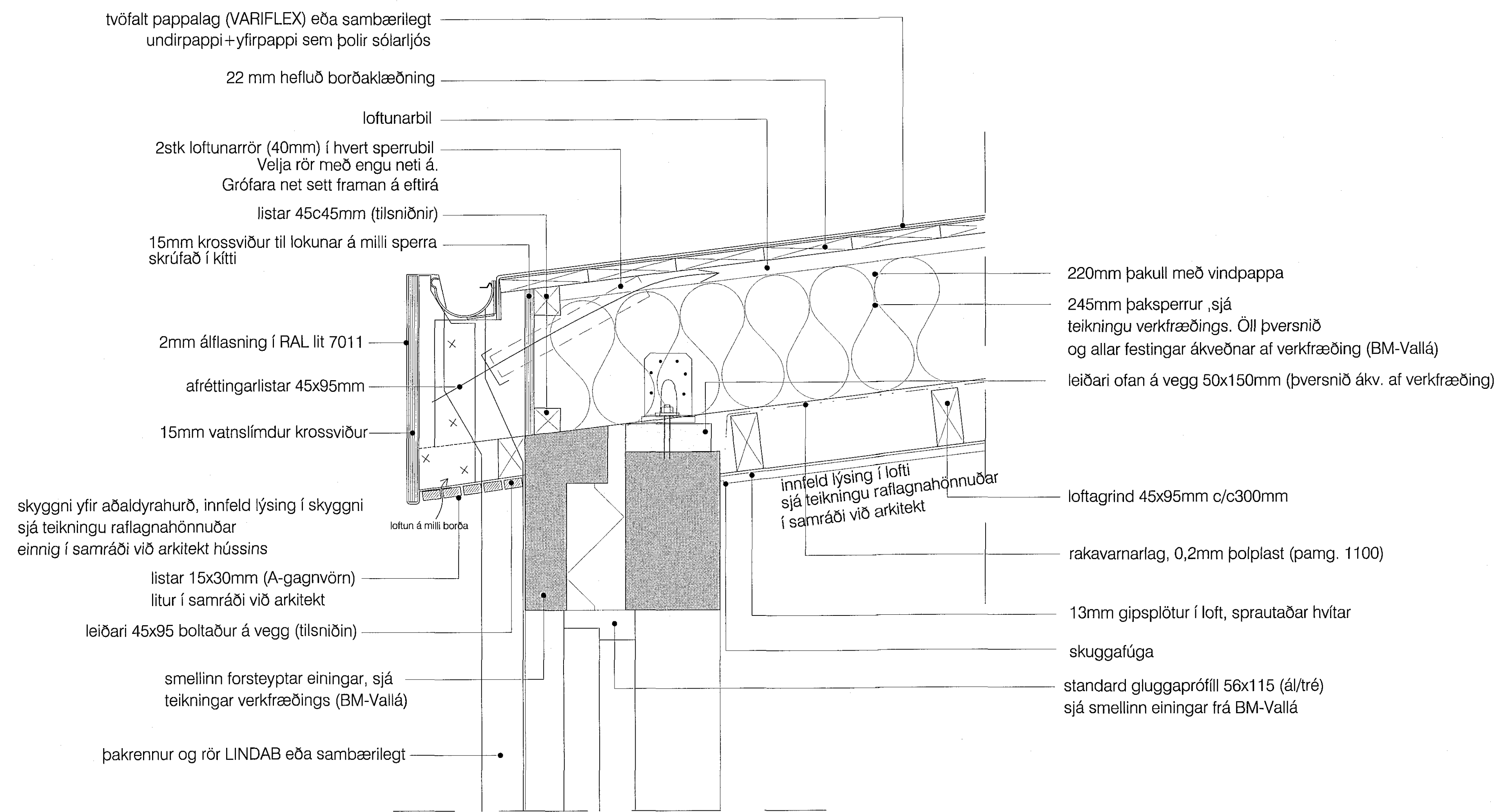
Deili 3-pakfrágangur (lóðrétt snið) styttri þakantur
