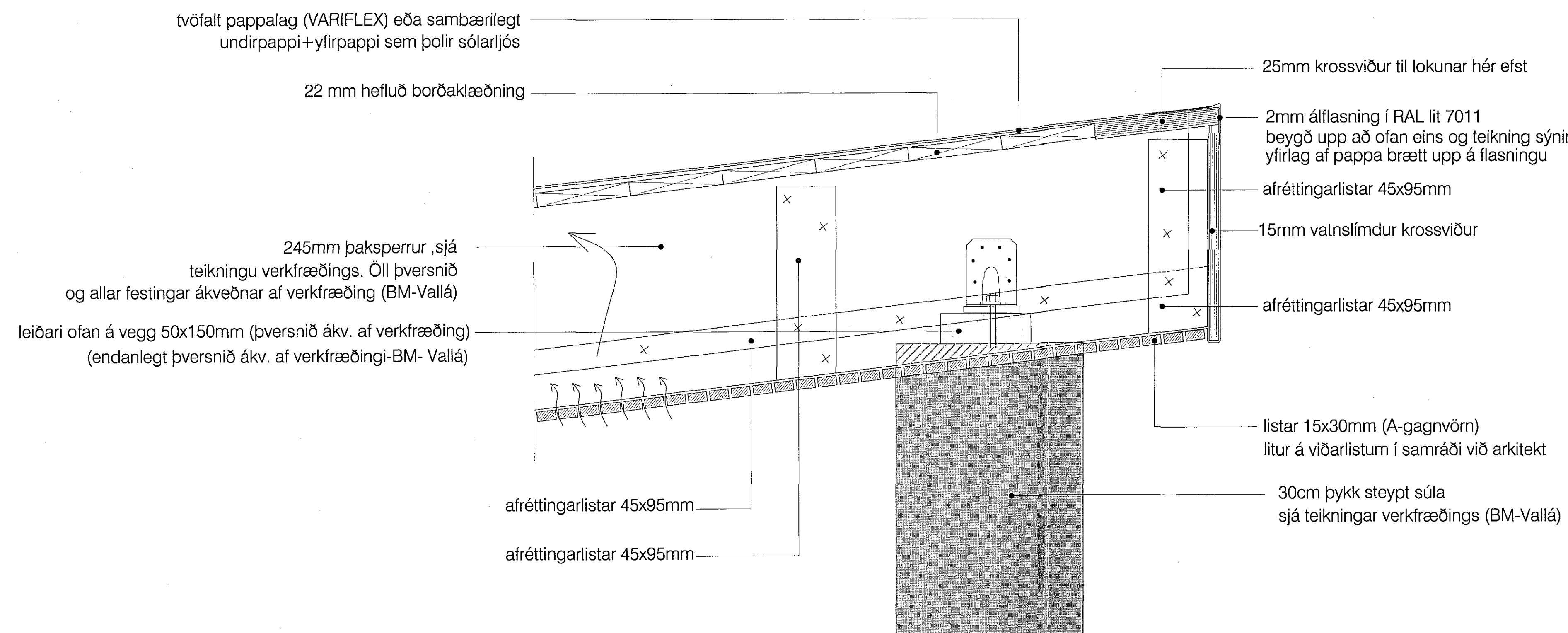
Deili 4-pakfrágangur (lóðrétt snið) þak yfir svölum (yfirbyggðar svalir)
