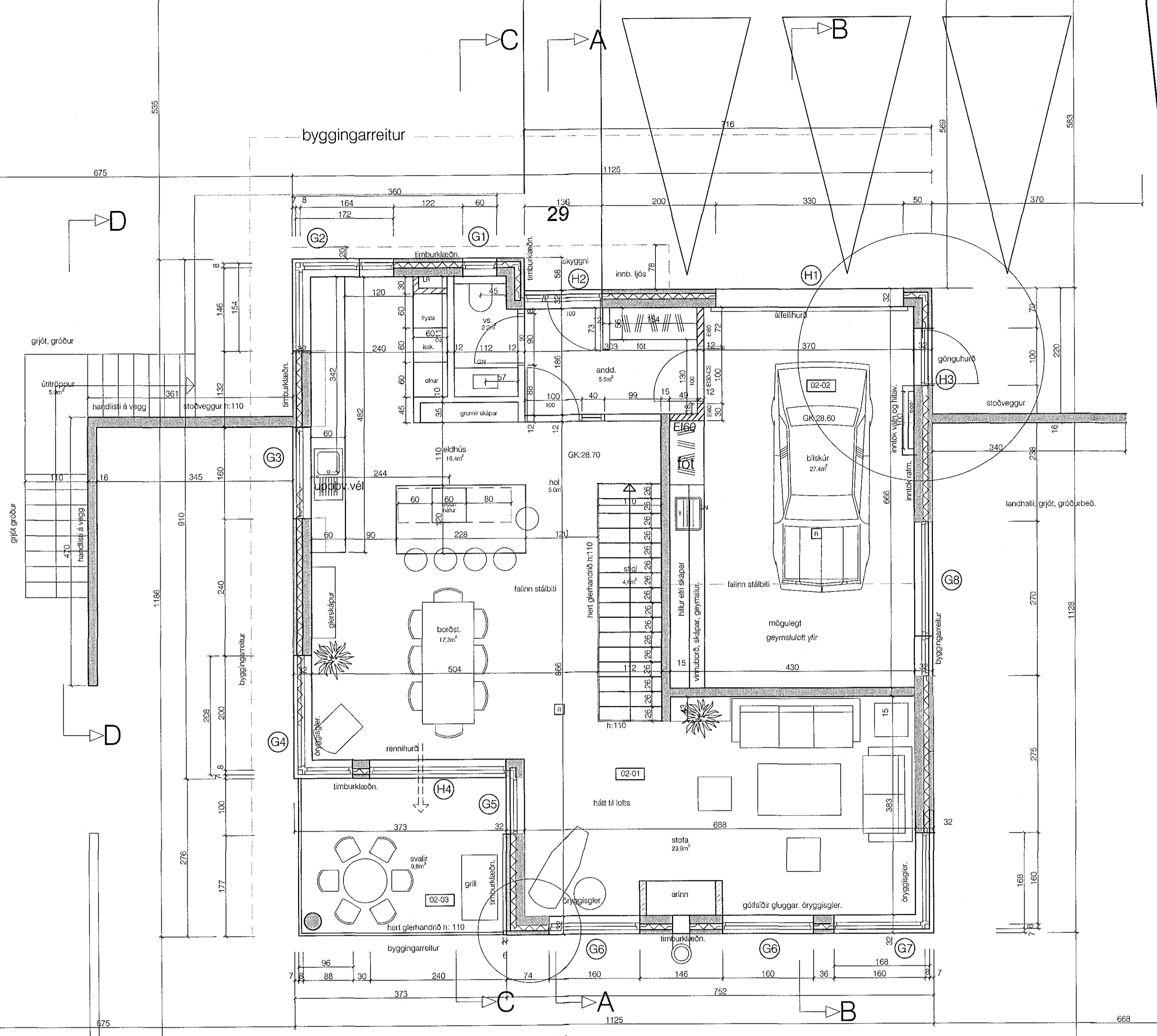
grunnmynd 2.hæð (götu-hæð)
