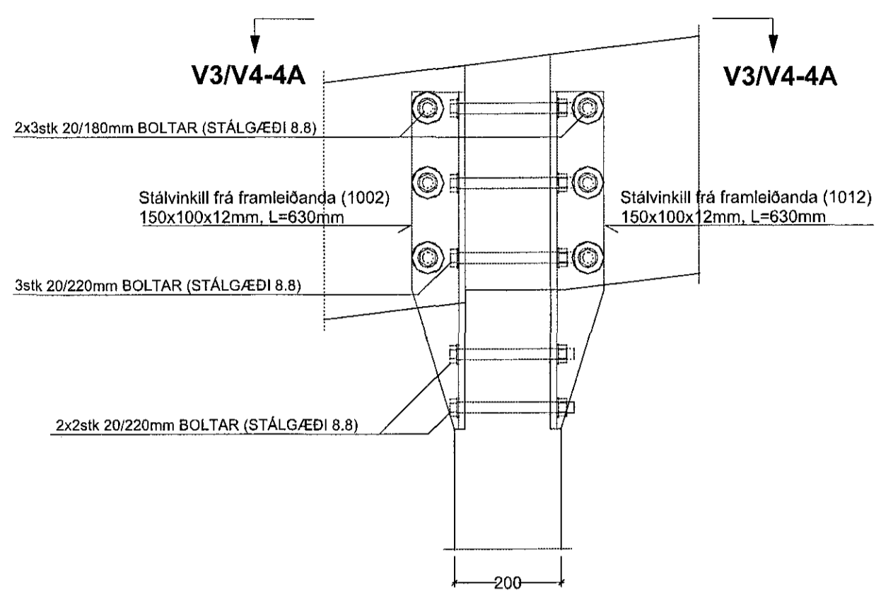
SNID V3/V4 - 4A MKV. 1:10
