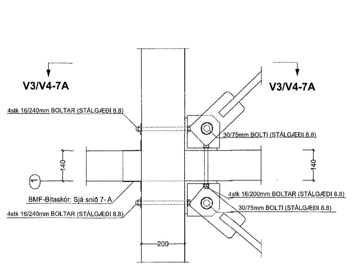
SNID V3/V4 - 7 MKV. 1:10
