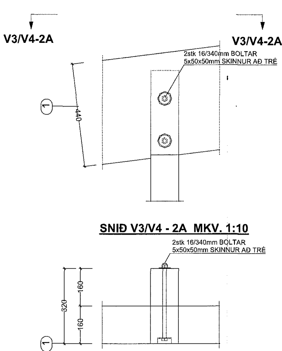
SNID V3/V4 - 2 MKV. 1:10
