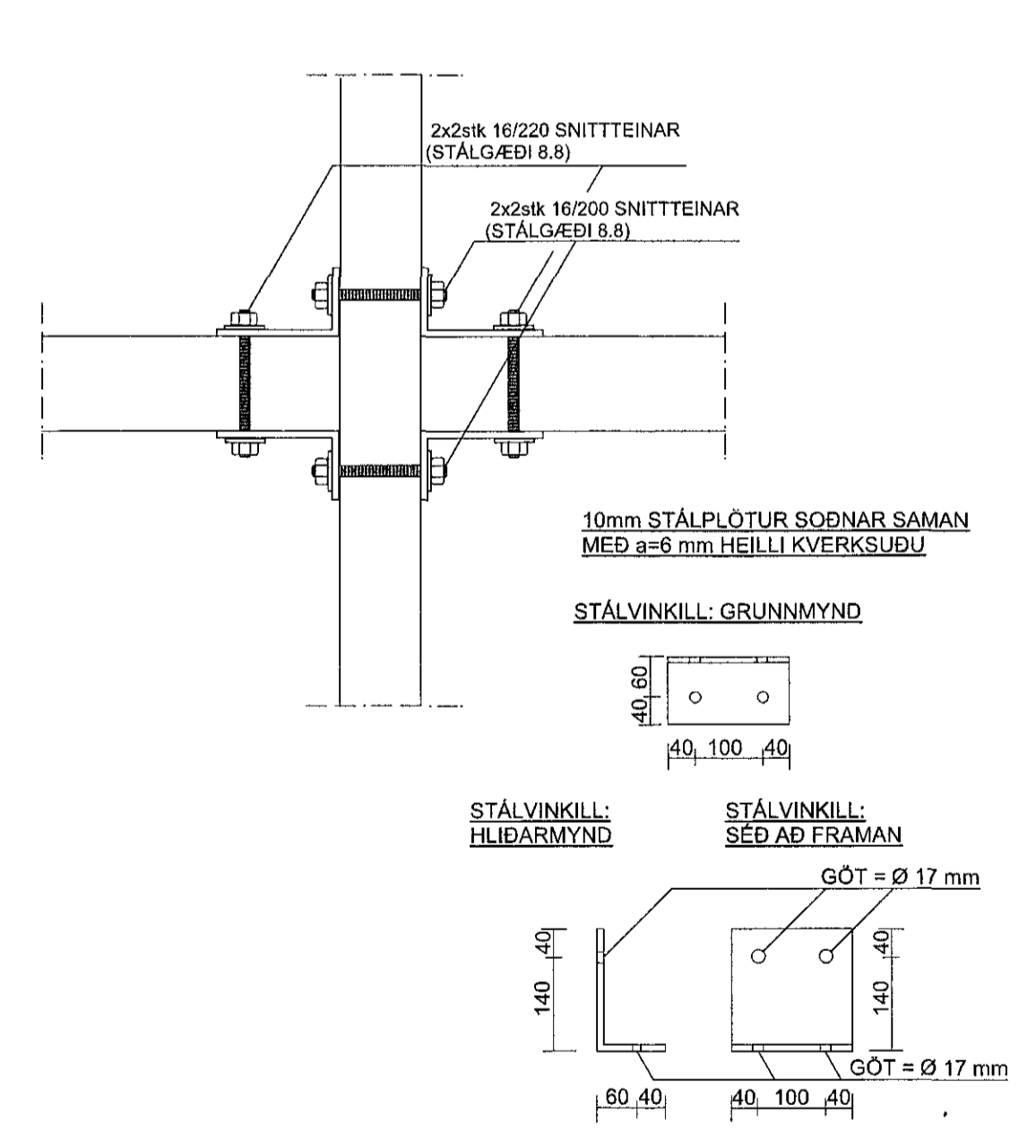
SNID V3/V4 - 9 MKV. 1:10
