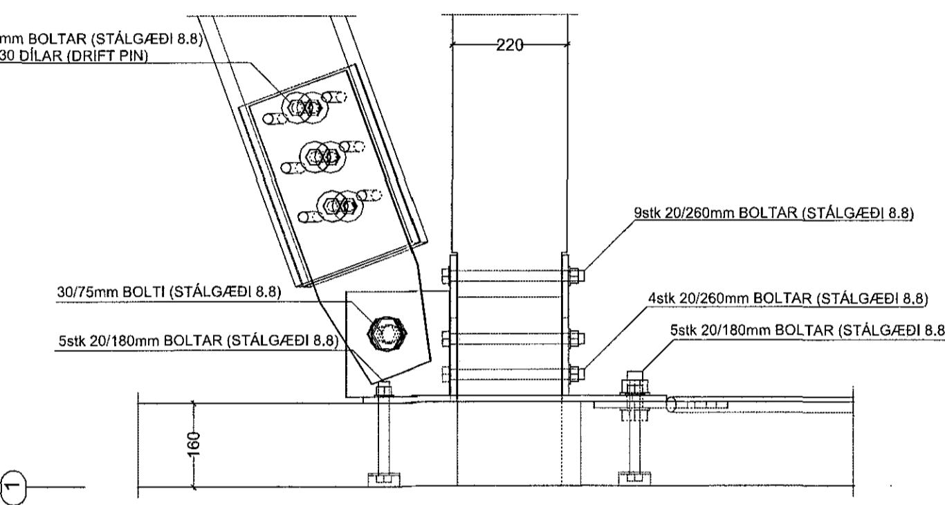
SNID V3/V4 - 7 MKV. 1:10
