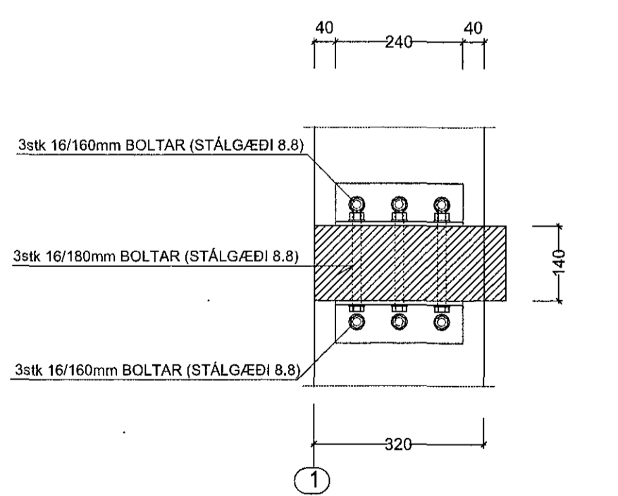
SNID V3/V4 - 8A MKV. 1:10
