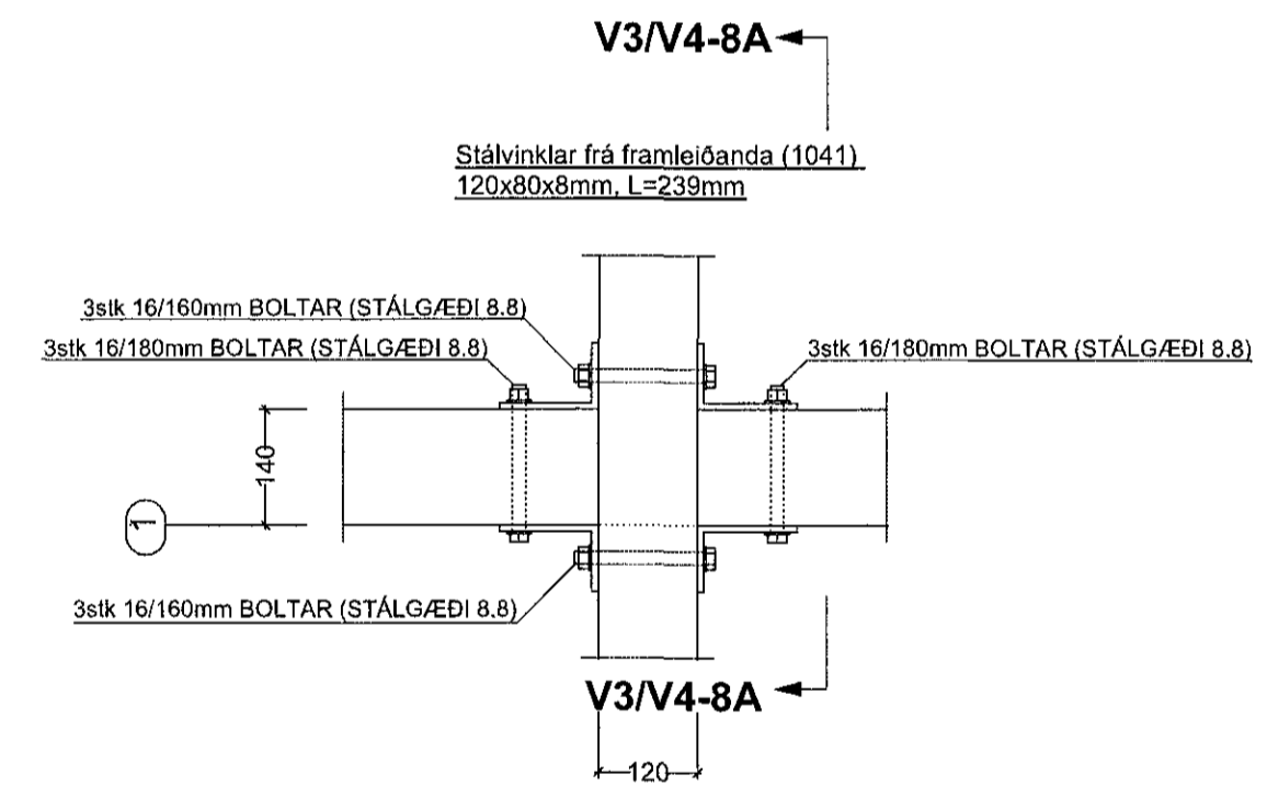
SNID V3/V4 - 8 MKV. 1:10
