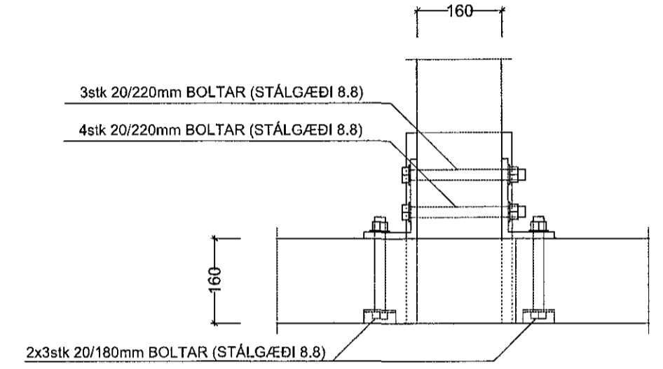
SNID V3/V4 - 4A MKV. 1:10
