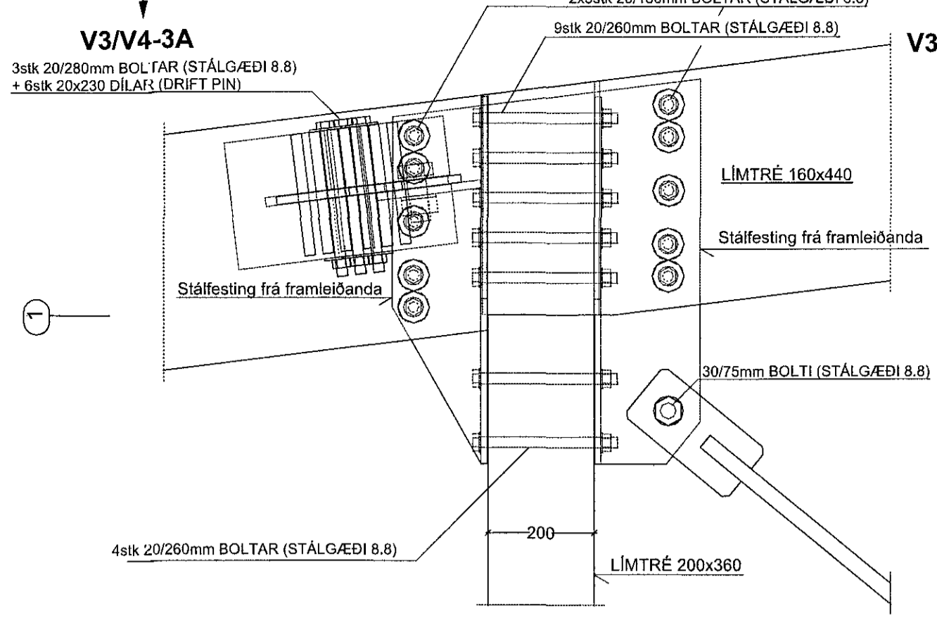
SNID V3/V4 - 3 MKV. 1:10
