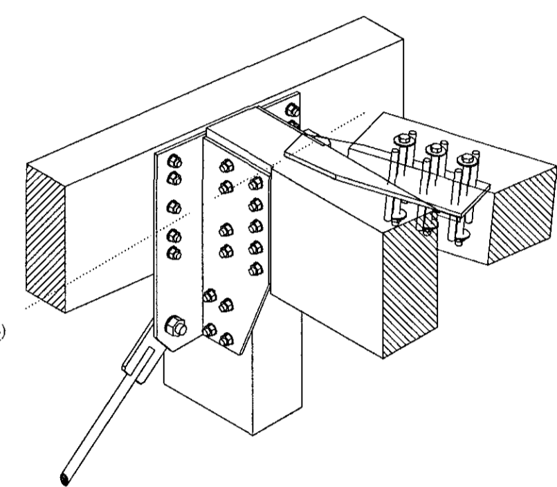
SNID V3/V4 - 3A MKV. 1:10 (Þrívíddarsjónarhorn af samsetningu)
