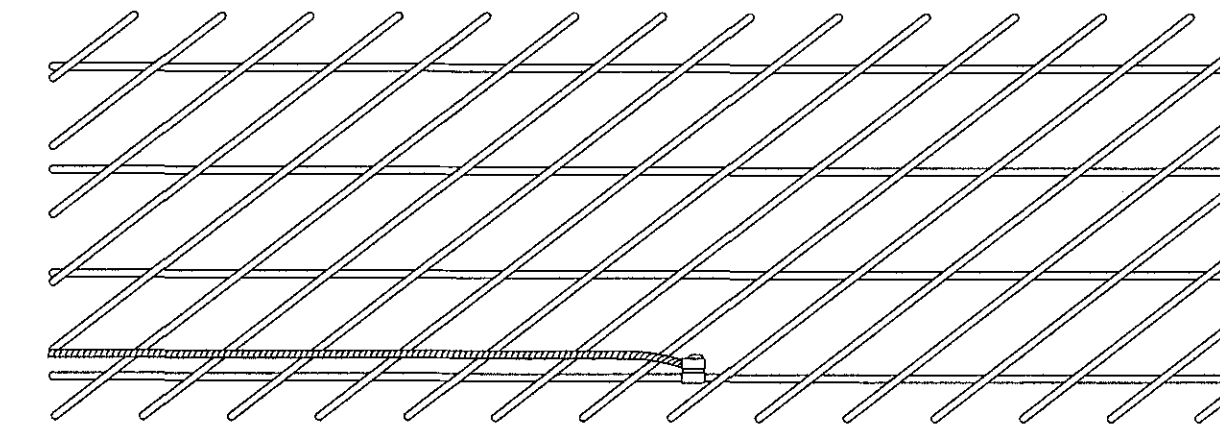
SÉRMYND E TENGINGAR JARÐTAUGA Í STEYPUSTRYKTARJÁRN
