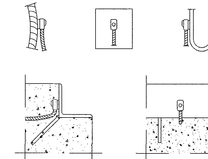
SÉRMYND F SODIN TENGING JARÐTAUGA Í STÁLRAMMA
