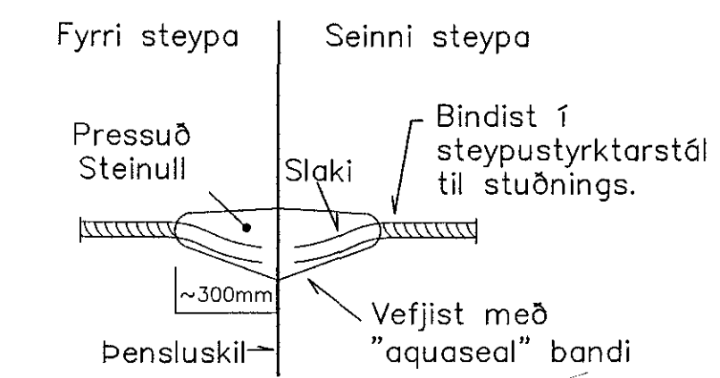
SÉRMYND G VERNDUN JARÐTAUGAR Á ÞENSLUSKILUM ÞAR SEM VIÐ A
