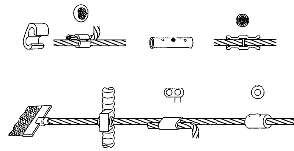
SÉRMYND A DÆMIGERÐAR TENGINGAR JARÐTAUGA ÓHEIMILT ER AÐ NOTA VIRALÁSA TIL TENGINGA JARÐTAUGA OG STEYPUJÁRN
