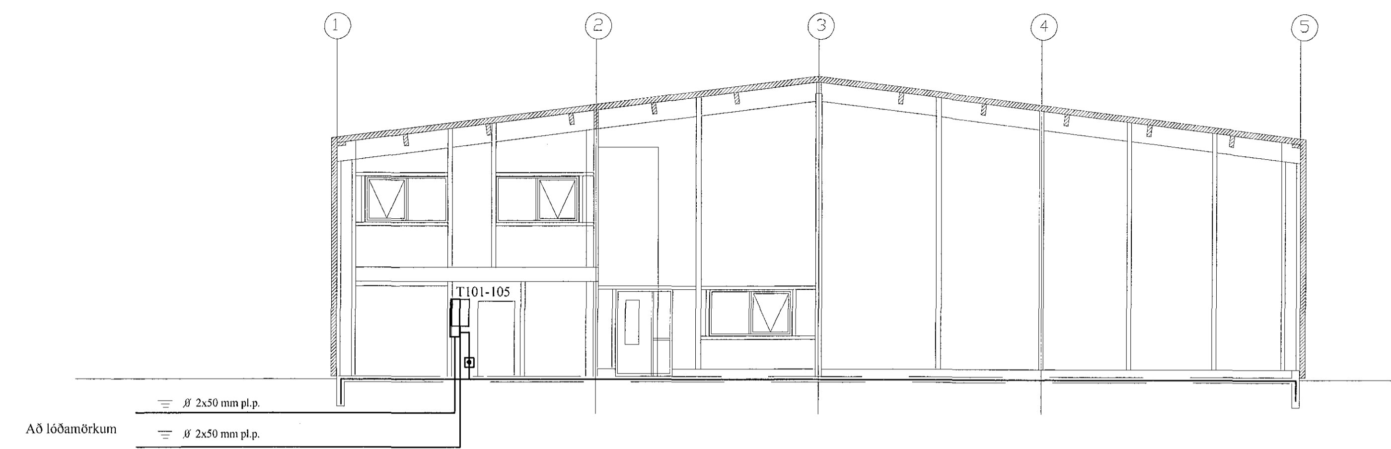
SNID Í INNTAK M 1:100
