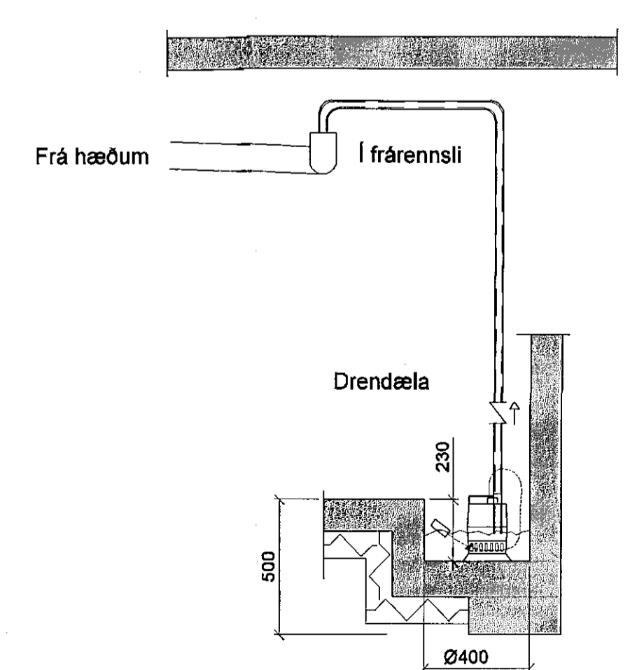
Drendæla (A-A) 1:20
