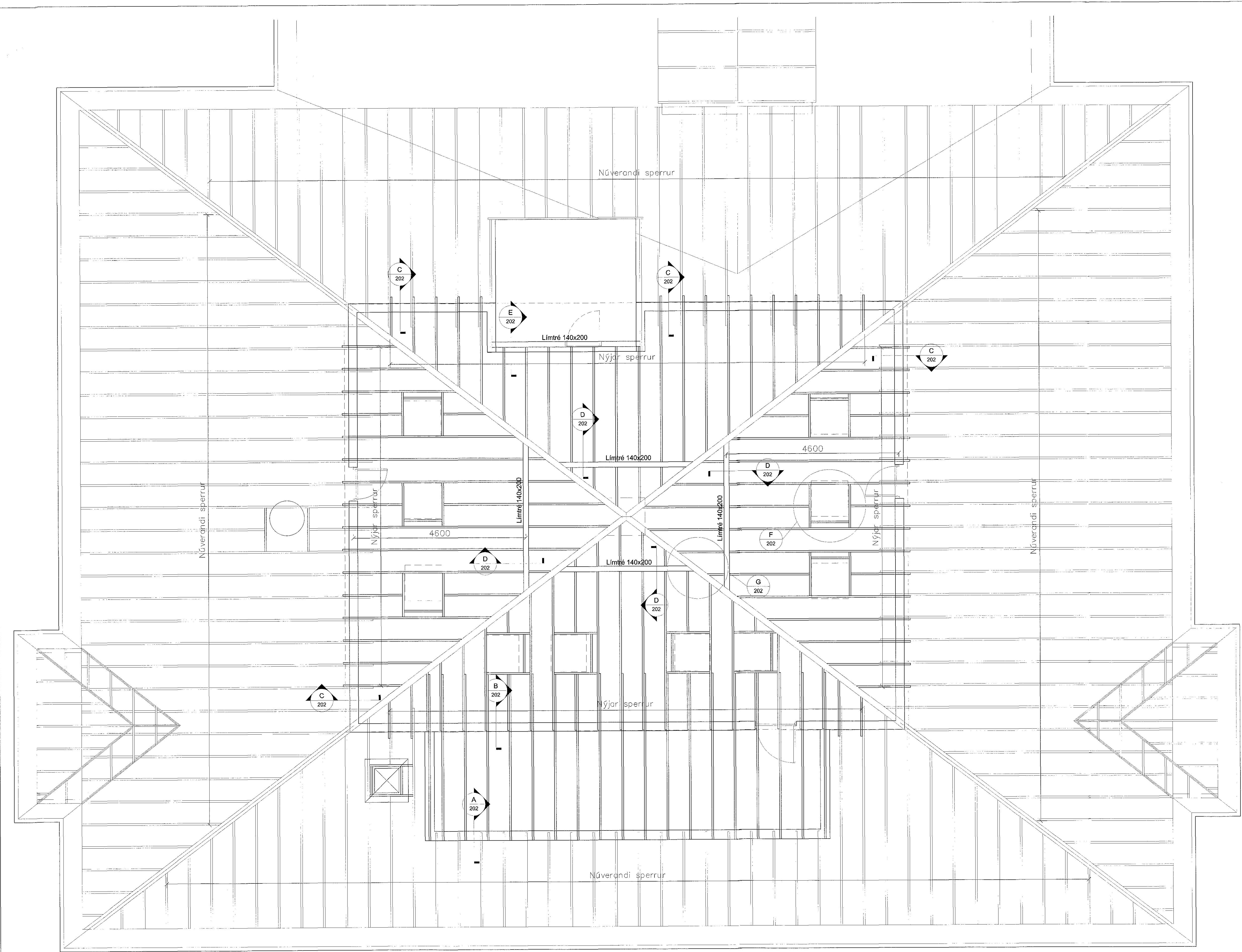
Grunnmynd af sperrum 1 = 50 mm
