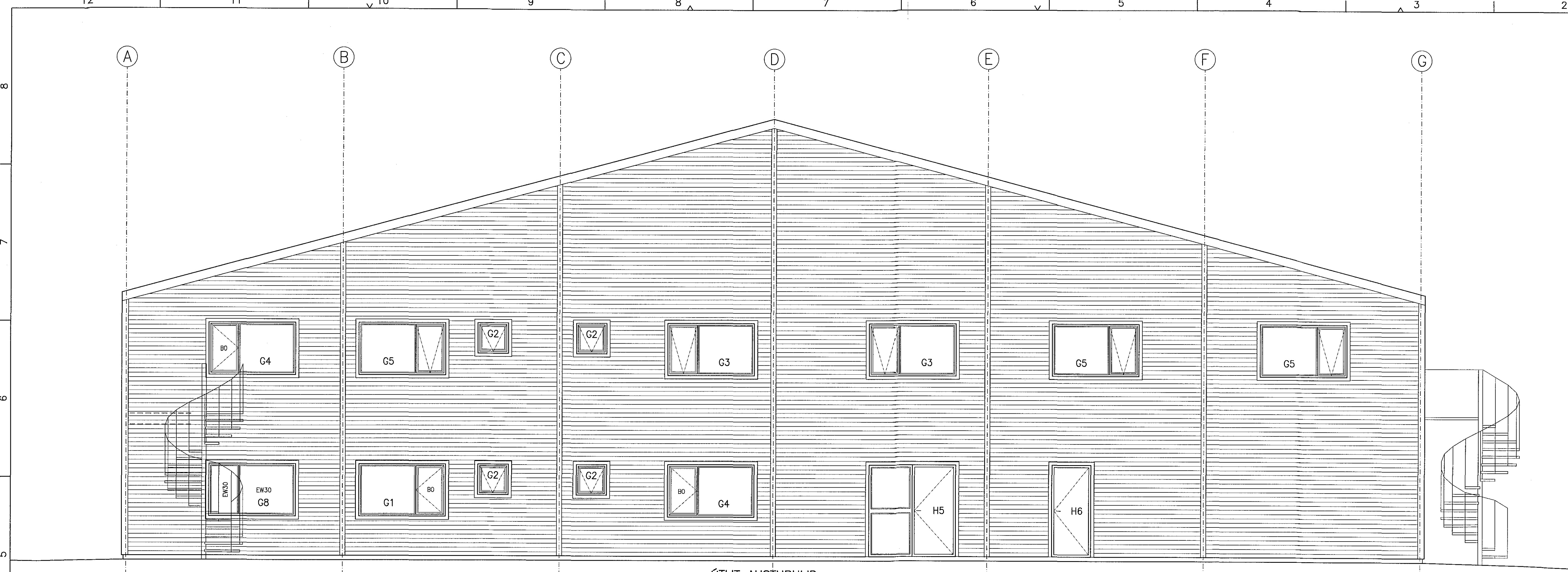
ÚTLIT AUSTURHLID
