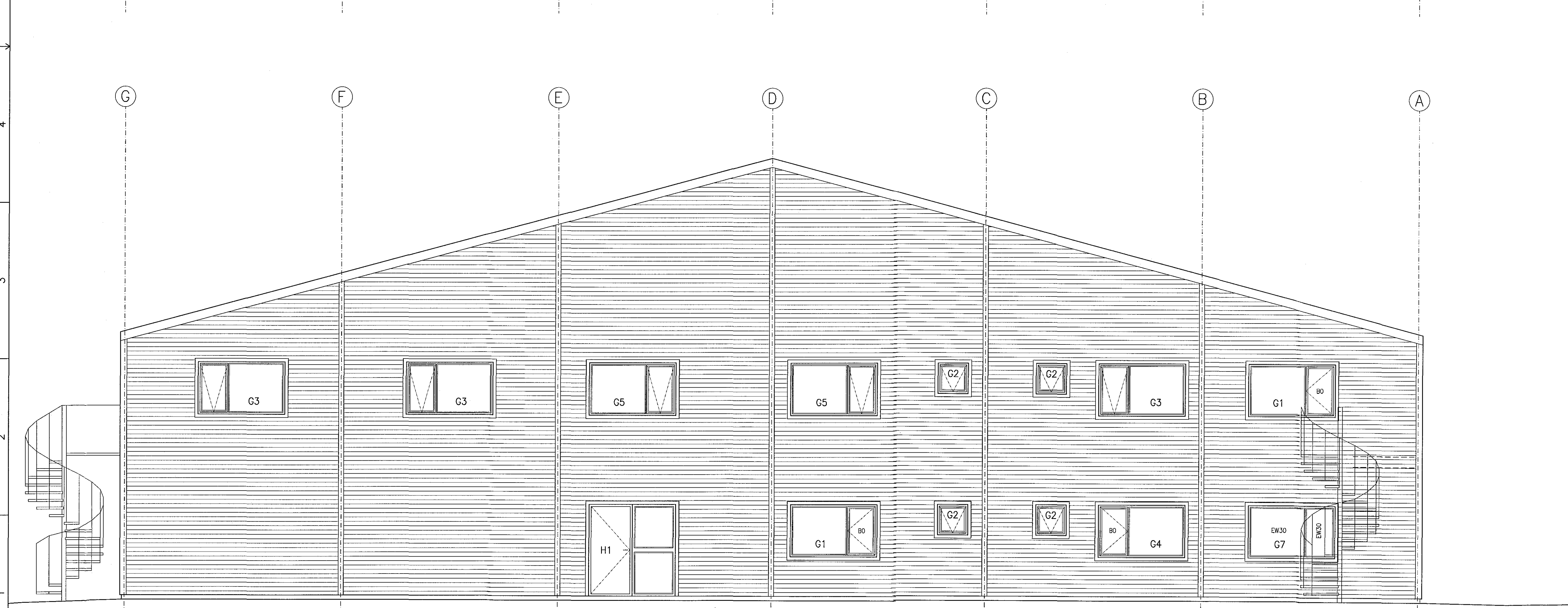
ÚTLIT VESTURHLID
