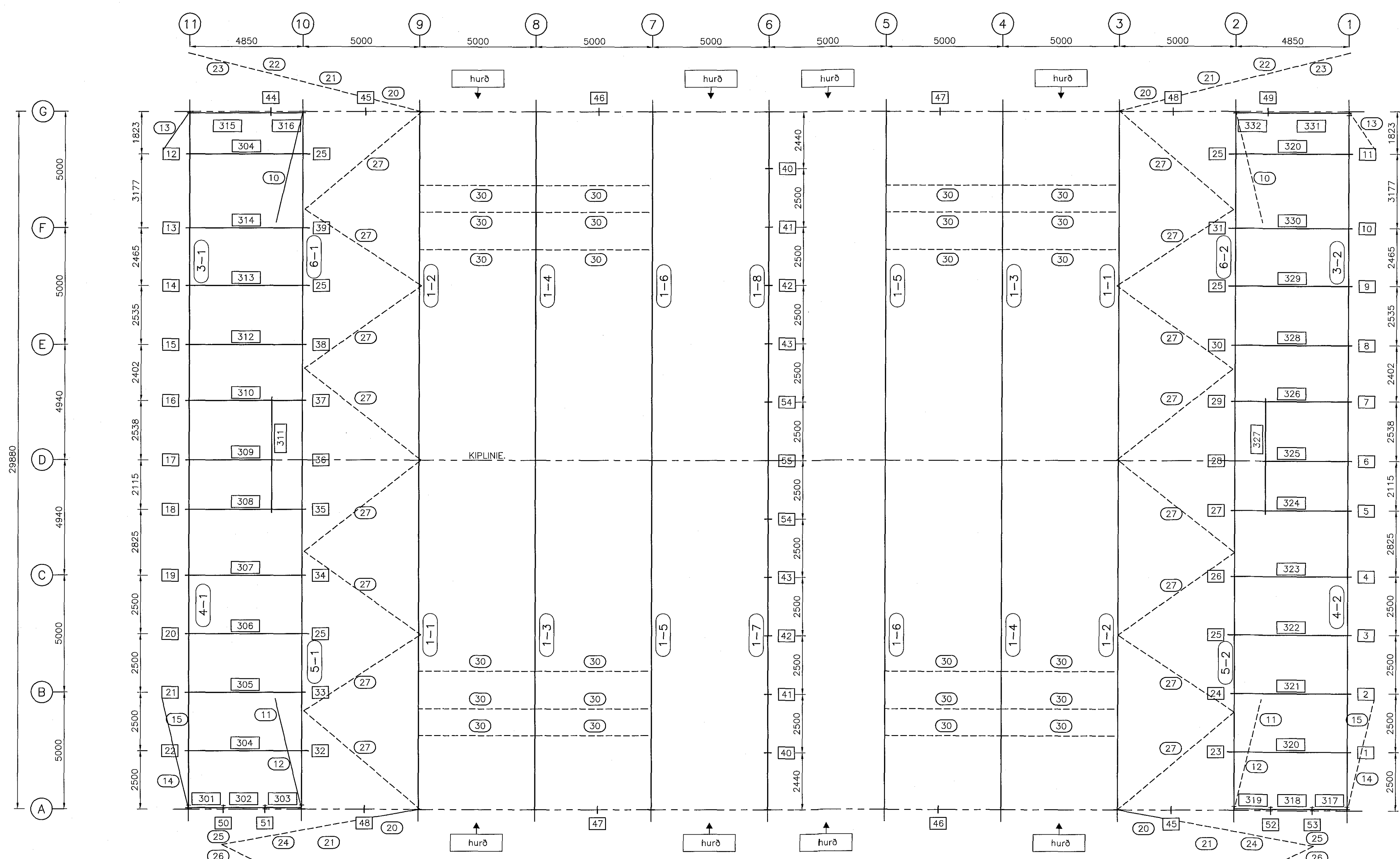
GRUNNMYND STÁLGRIND 1:100
