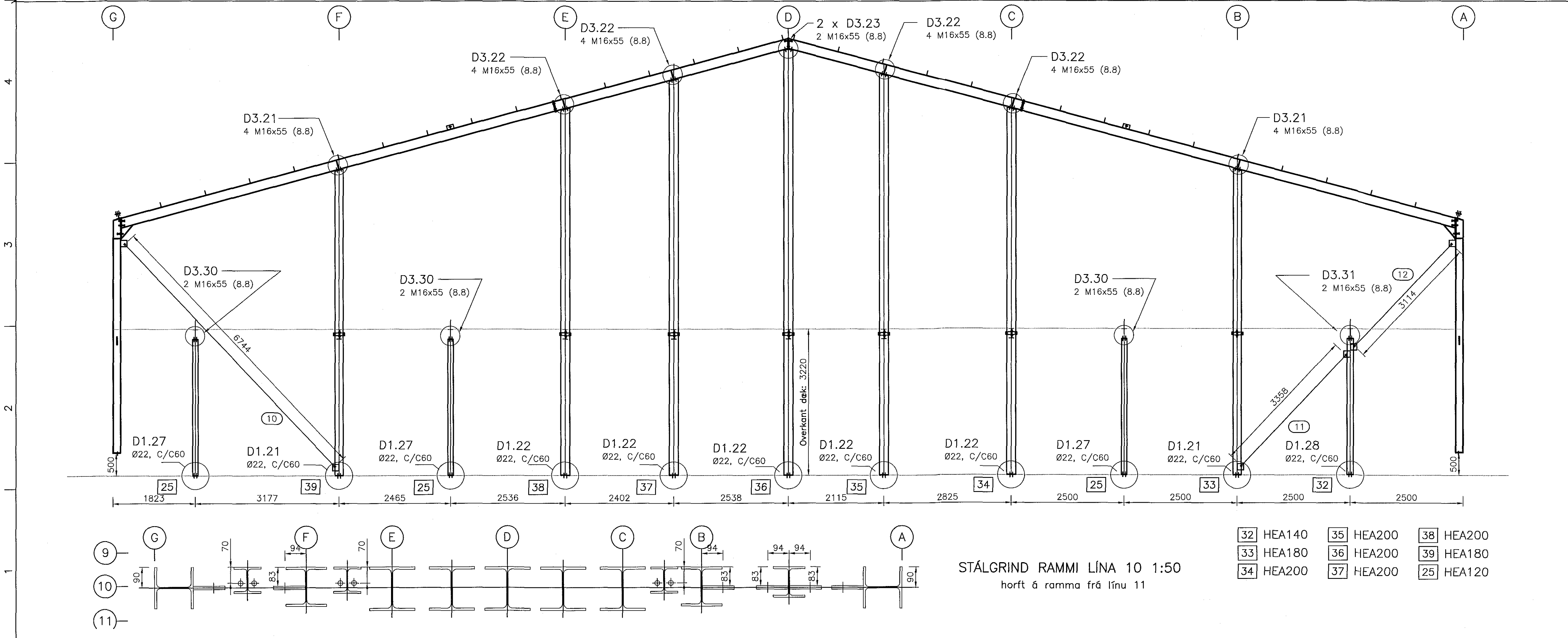
STÁLGRIND RAMMI LÍNA 6 1:50 horft á ramma frá línu 7
