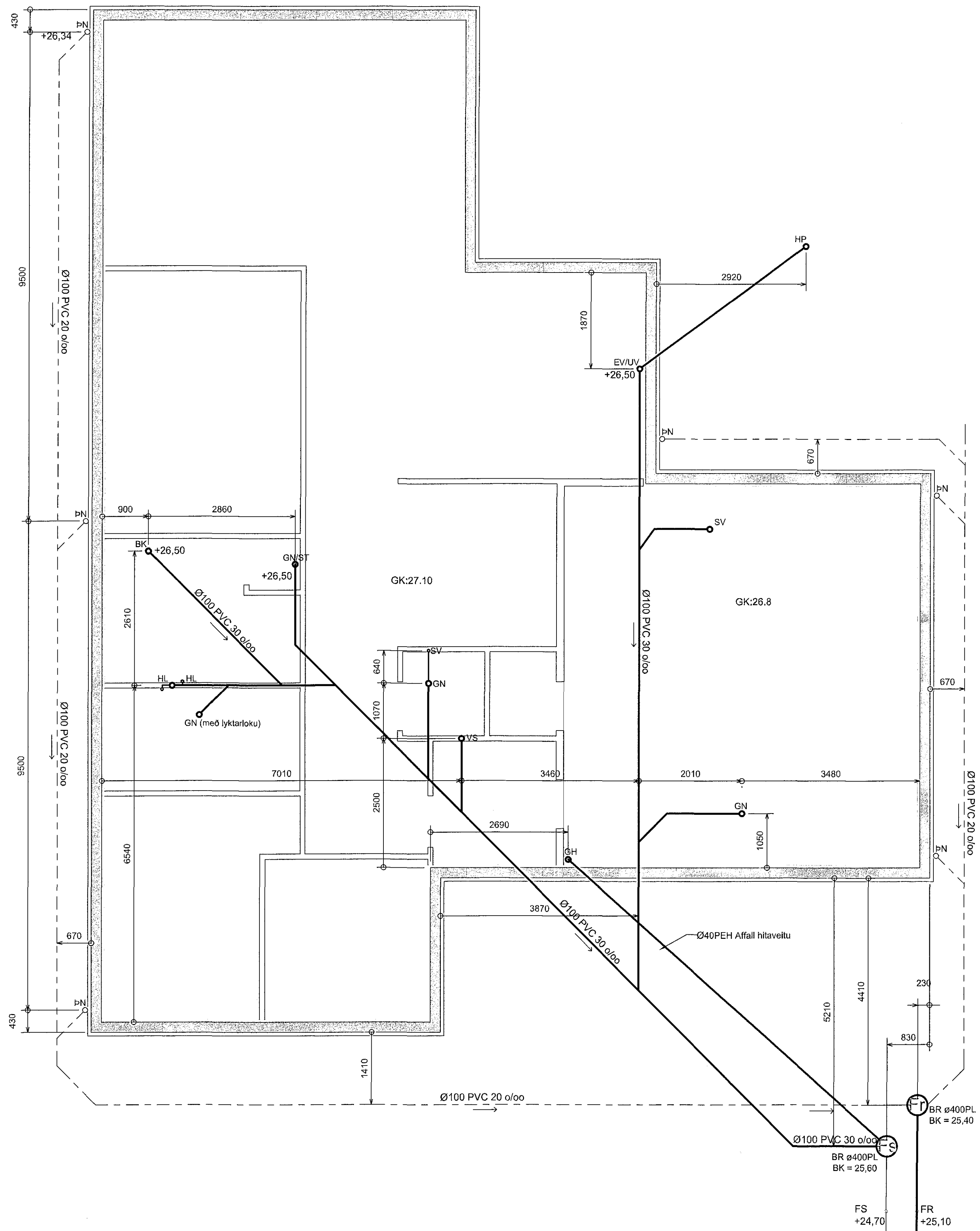
GRUNNMYND FRÁRENNSLI MKV. 1:50
