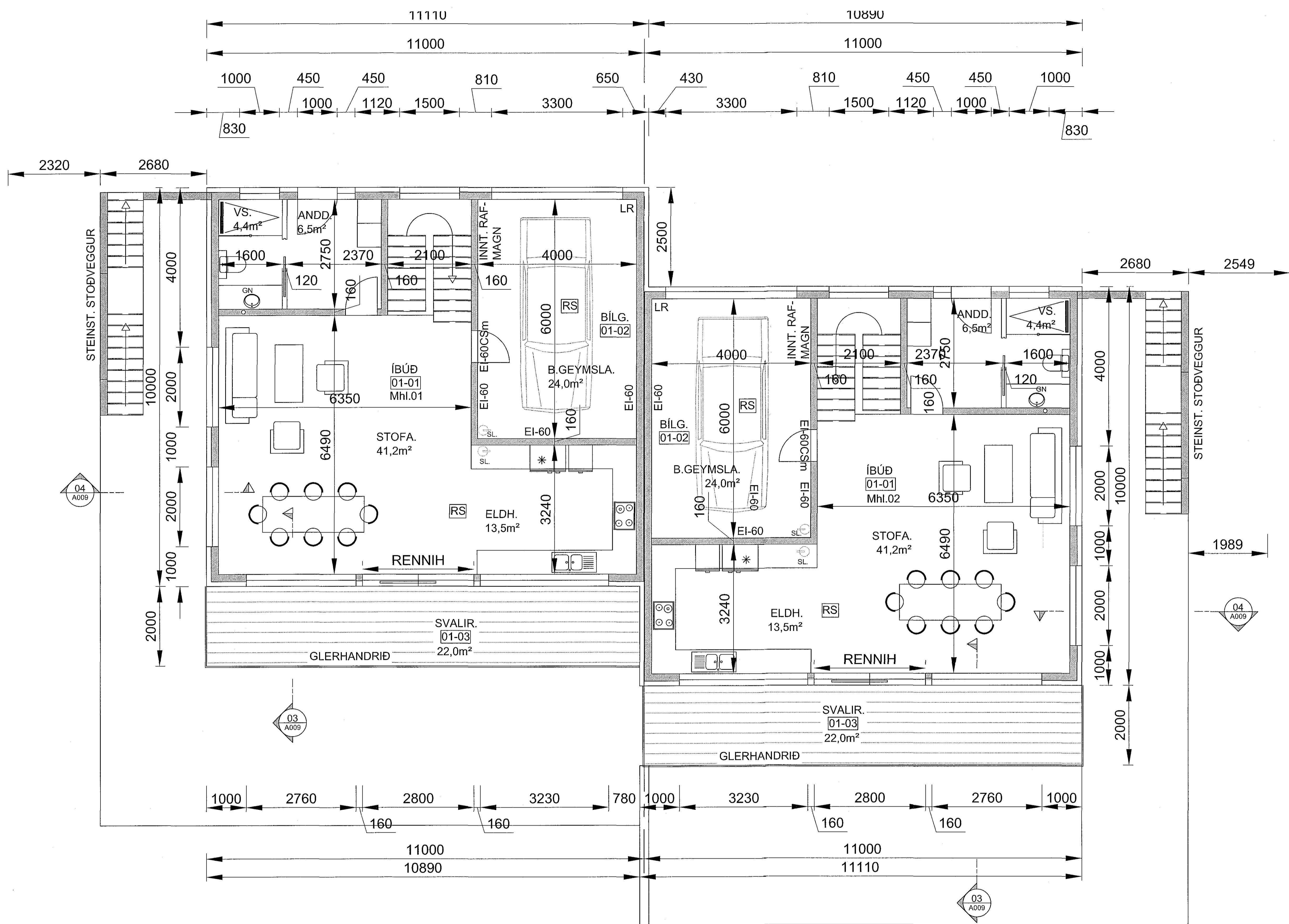
GRUNNMYND 1.HÆÐ 1:50 (A1)
