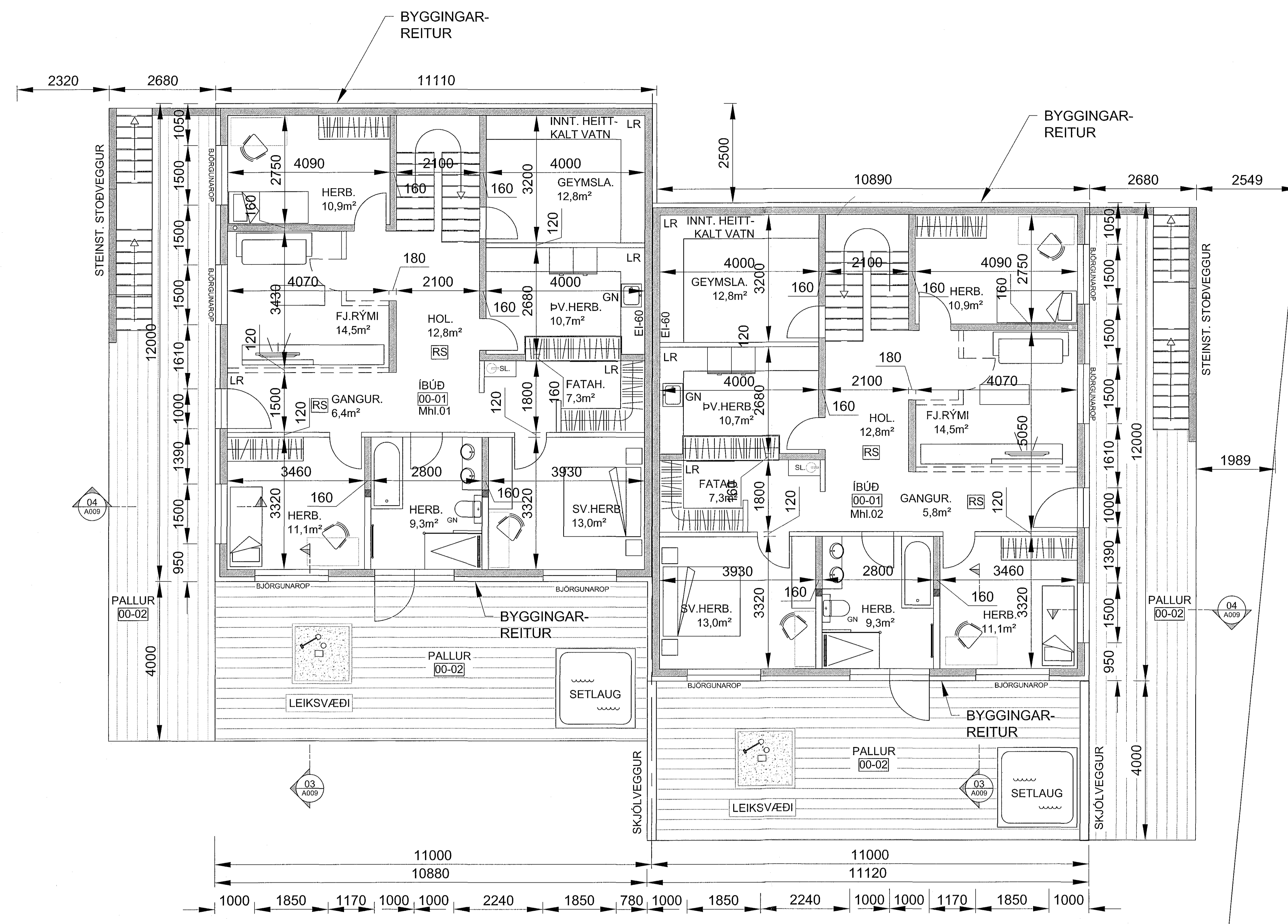
GRUNNMYND KJALLARI 1:50 (A1)
