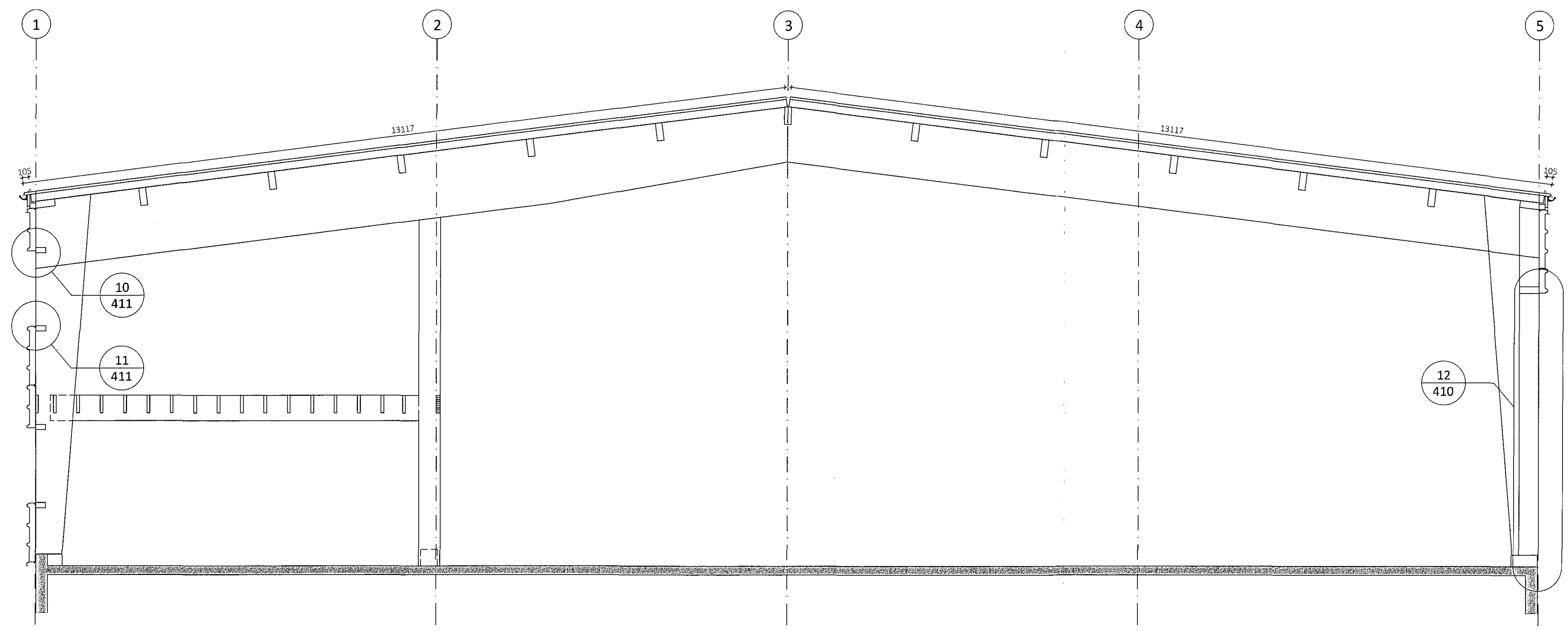
Þversnið A Mkv. 1:50 401
