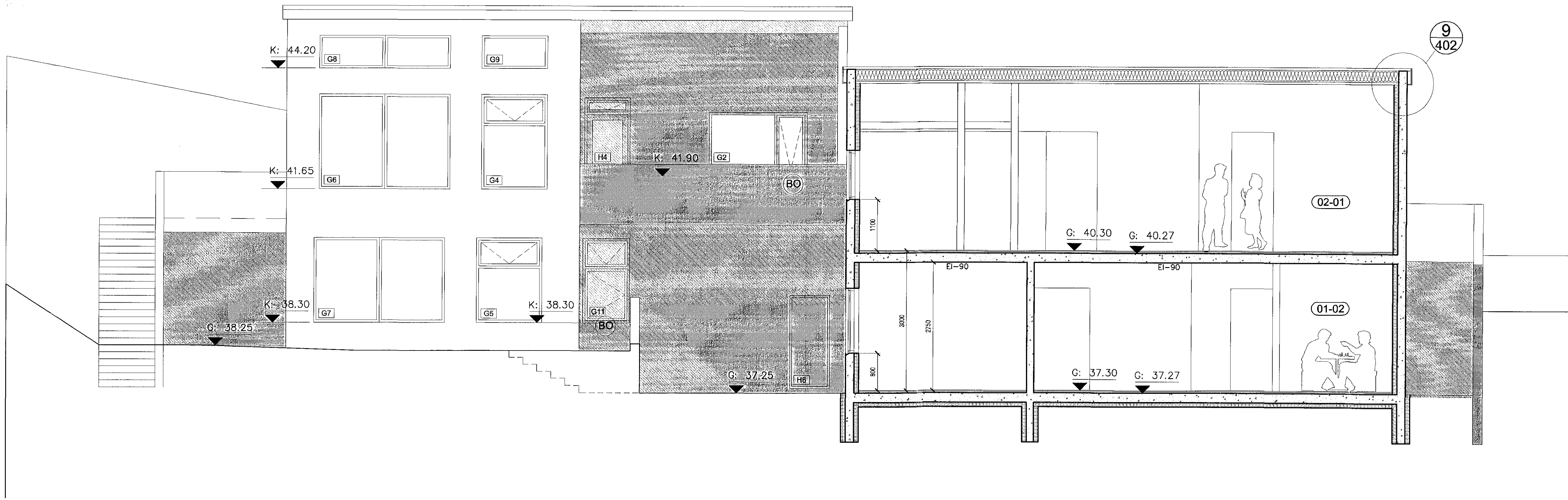
Sneiðing EE mkv. 1:50
