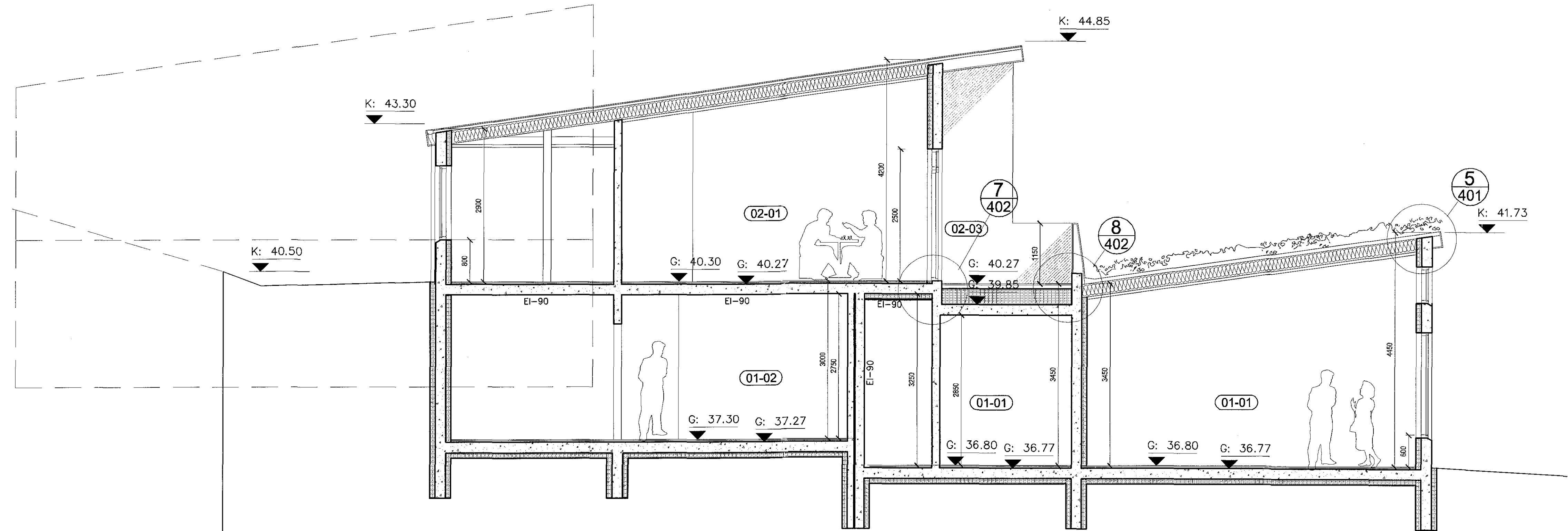
Sneiðing DD mkv. 1:50
