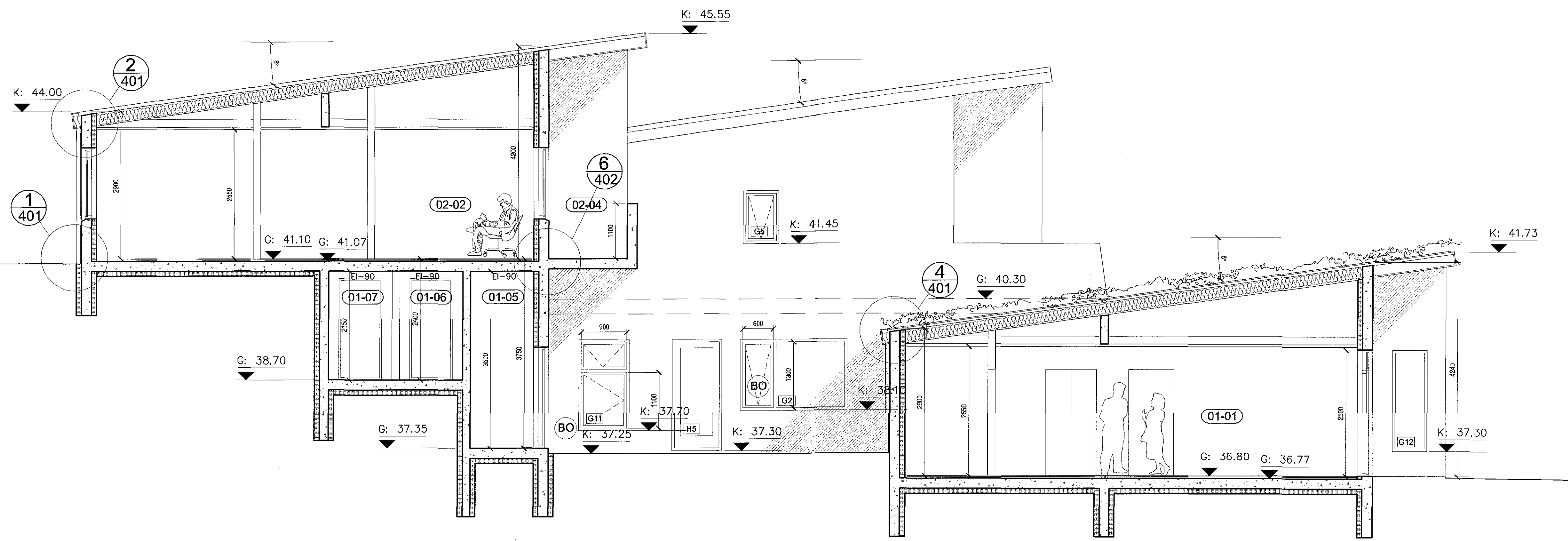
Sneiðing CC mkv. 1:50
