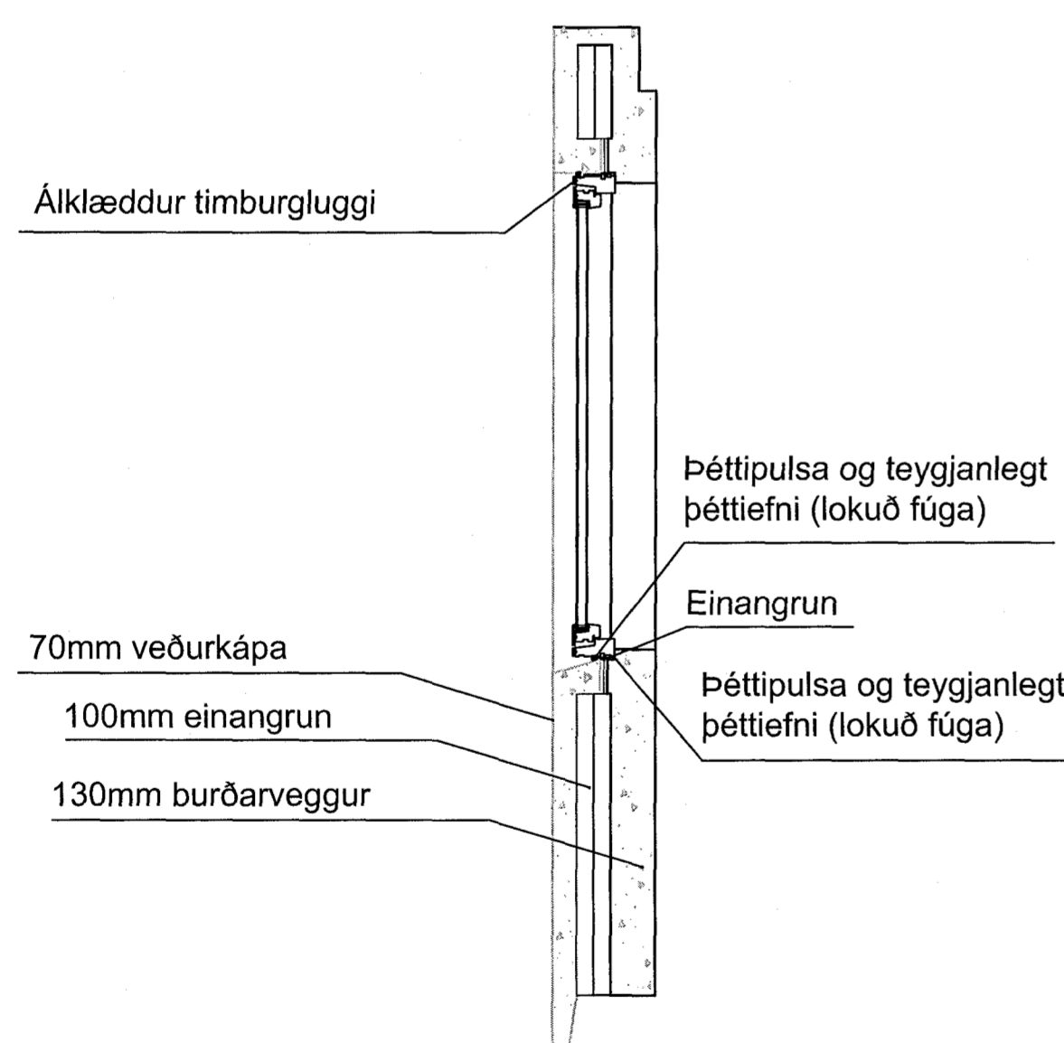
GD-001 Mkv. 1:20 Allmenur frágangur glugga
