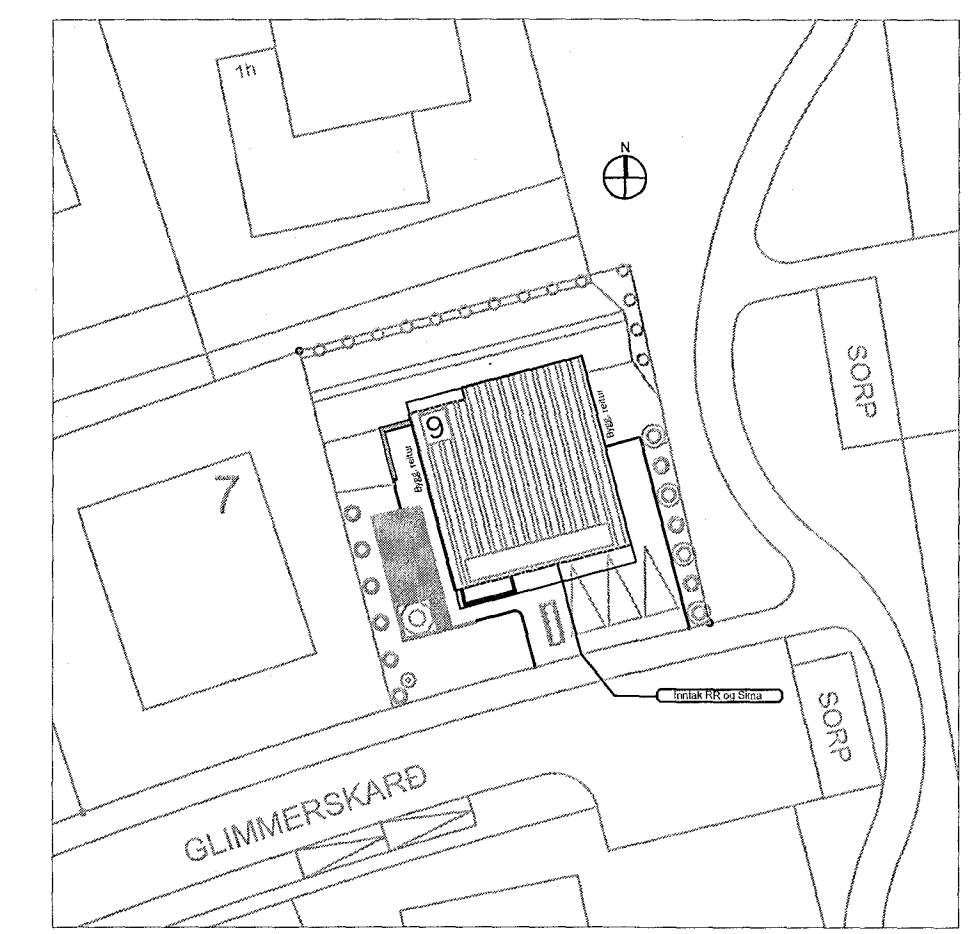
Mvk 1:500
