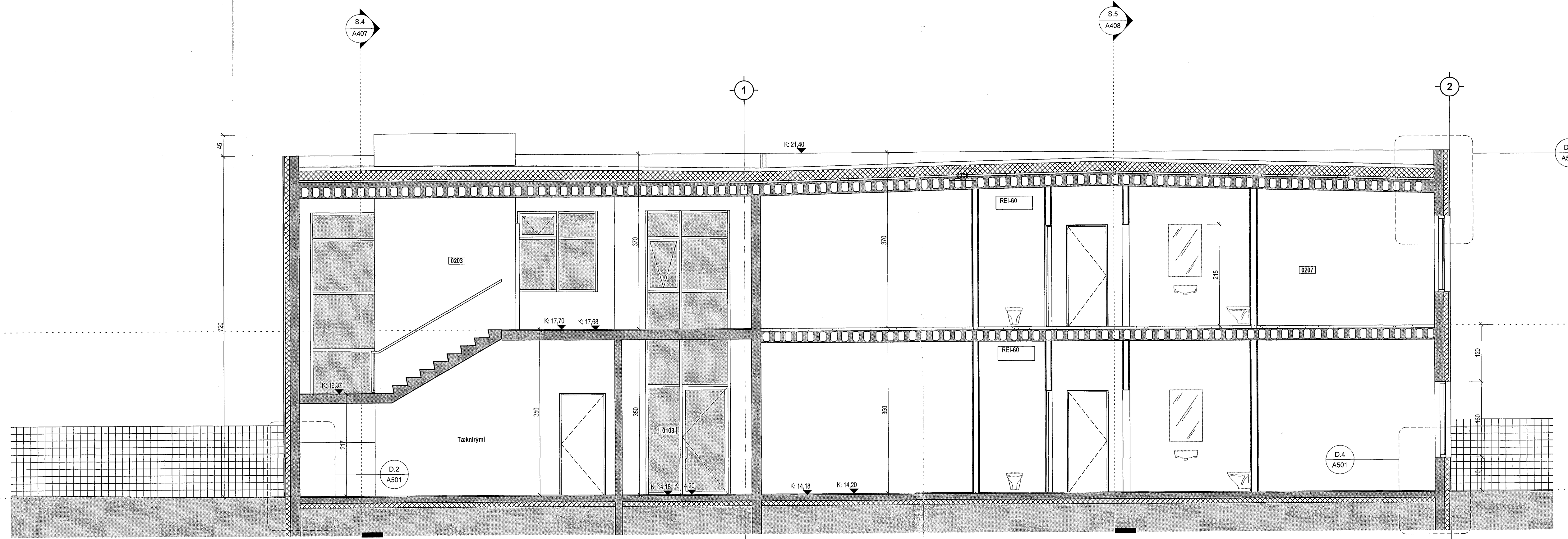
Snið 2 1:50
