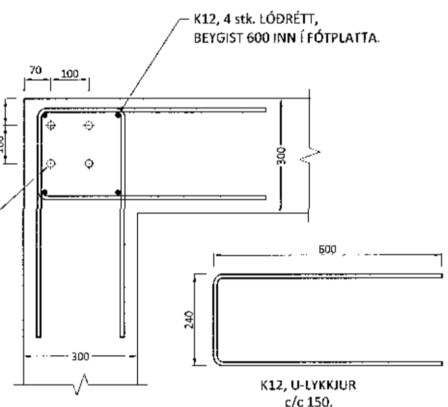
DEILI (D1) 1:10
