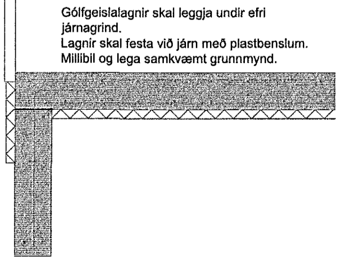
Staðsetning hitalagna í gólf M 1:20
