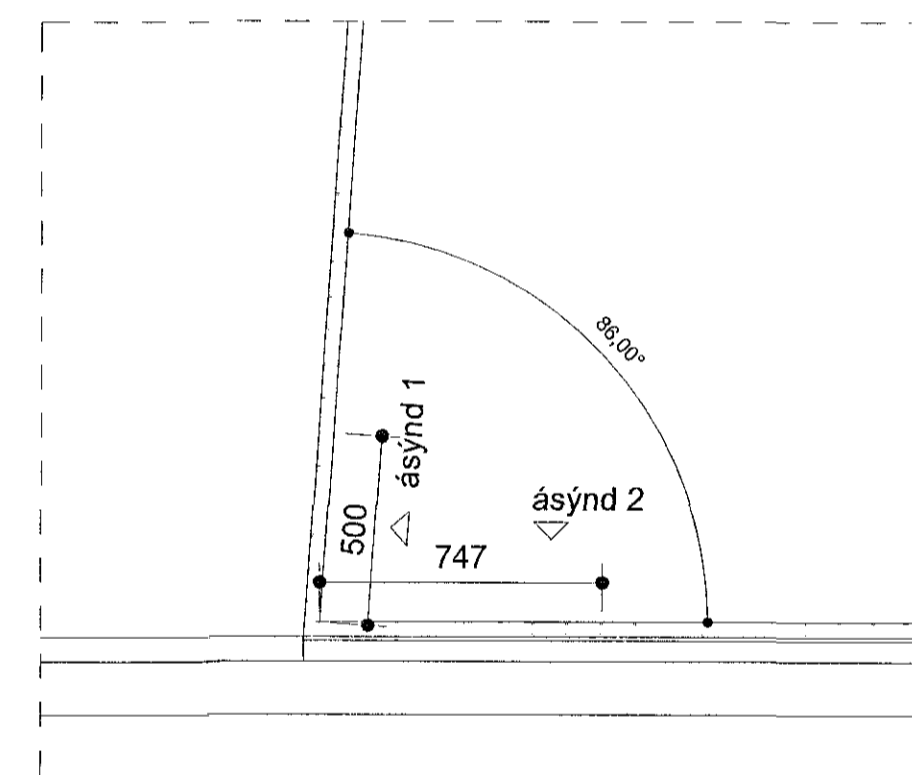
Svalahandrið 01_Hluti 7_grunnmynd mkv: 1 : 20
