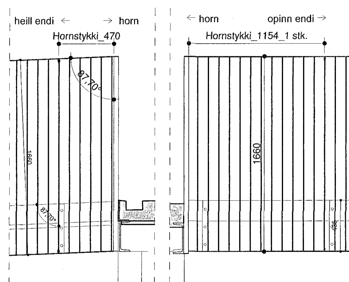
Hluti 5 ásýnd 1 mkv: 1 : 20 Hluti 5 ásýnd 2 mkv: 1 : 20
