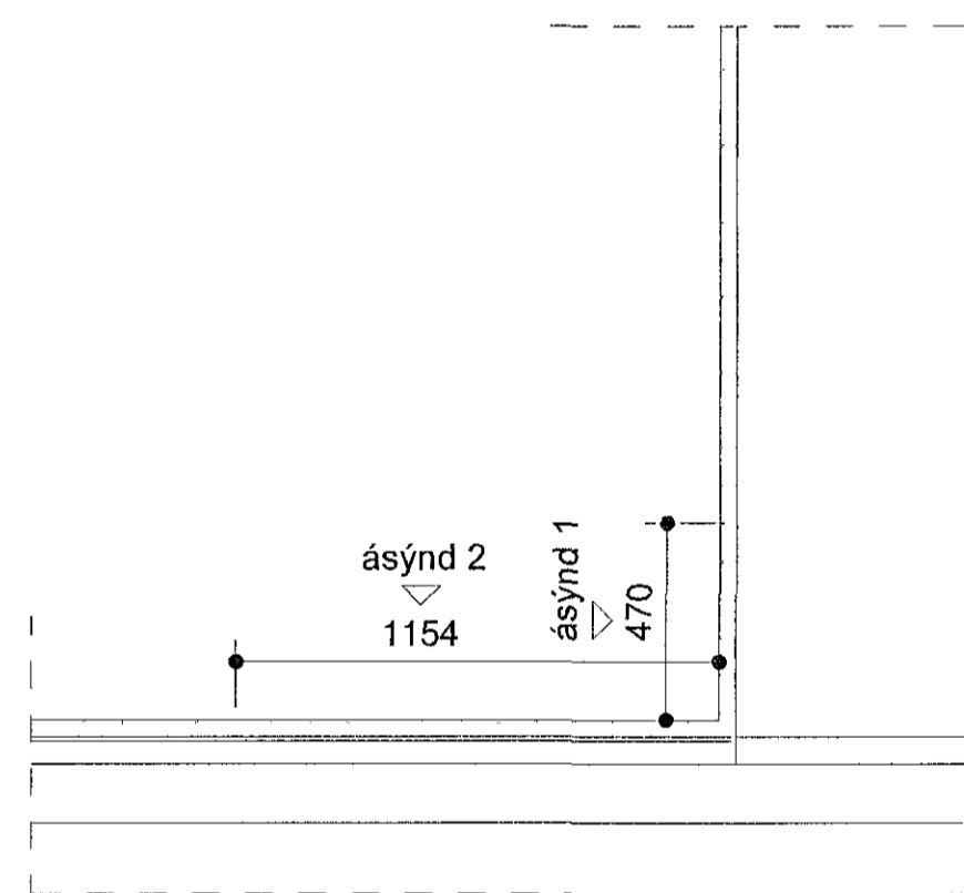
Svalahandrið 01_Hluti 5_grunnmynd mkv: 1 : 20
