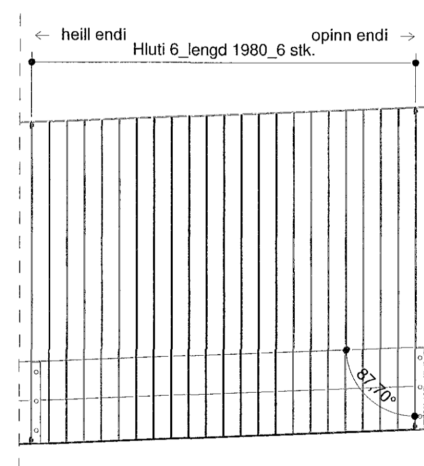
Hluti 6 ásýnd mkv: 1 : 20
