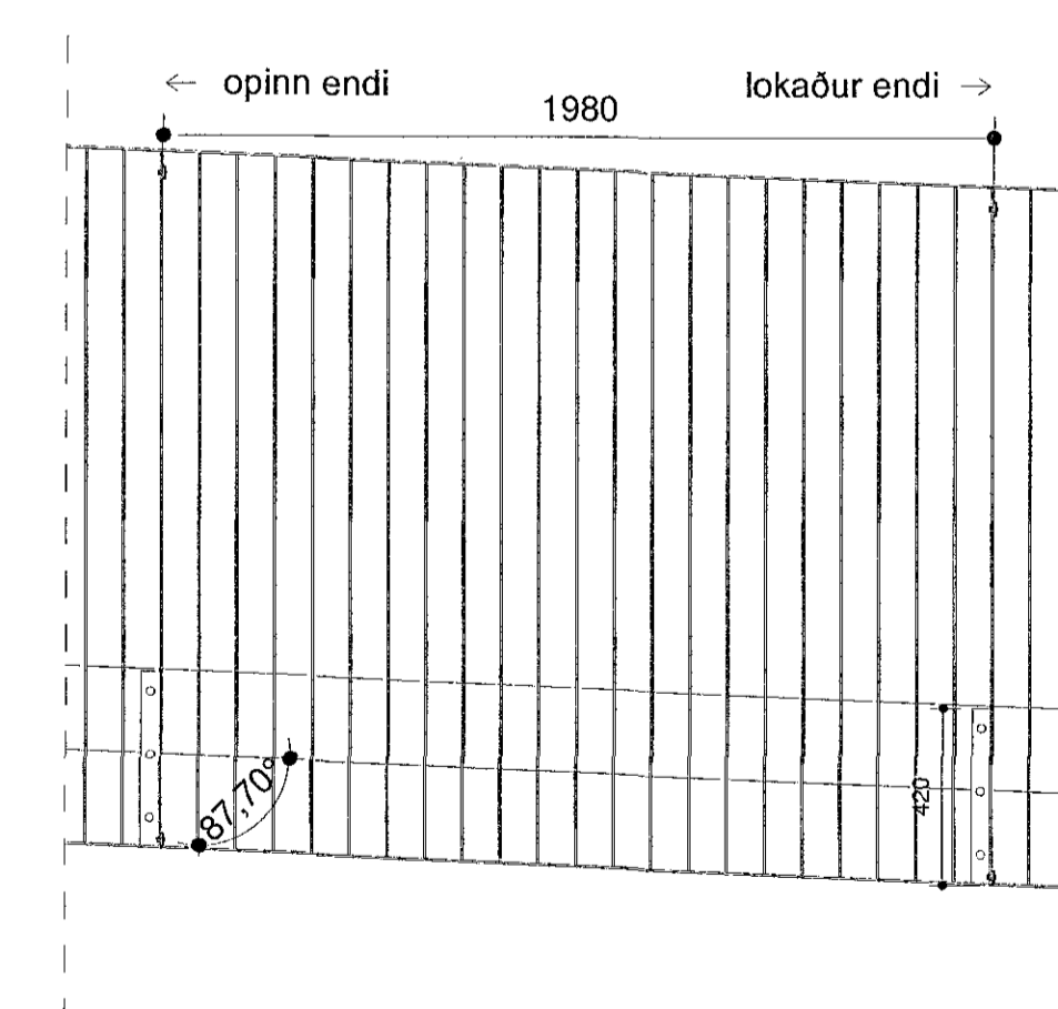
Hluti 8 ásýnd mkv: 1 : 20
