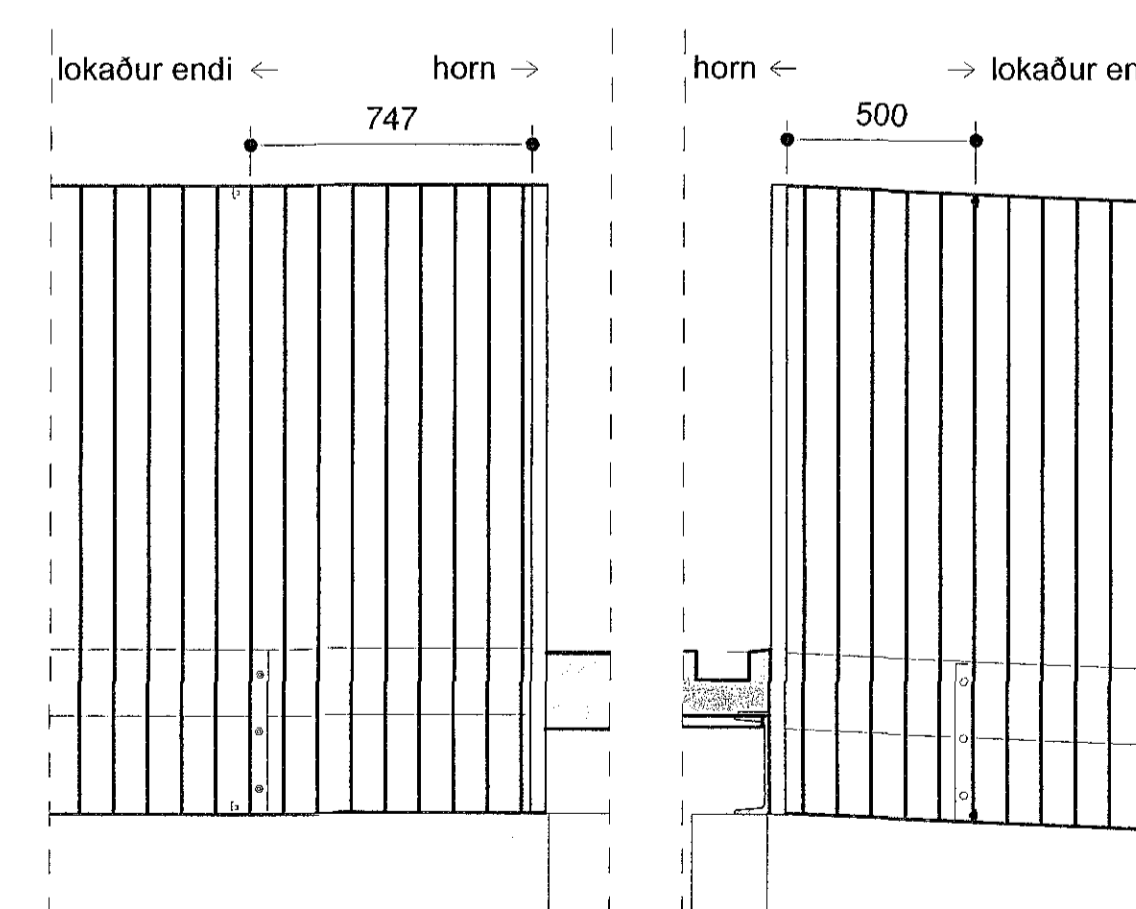
Hluti 7 ásýnd 1 mkv: 1 : 20 Hluti 7 ásýnd 2 mkv: 1 : 20
