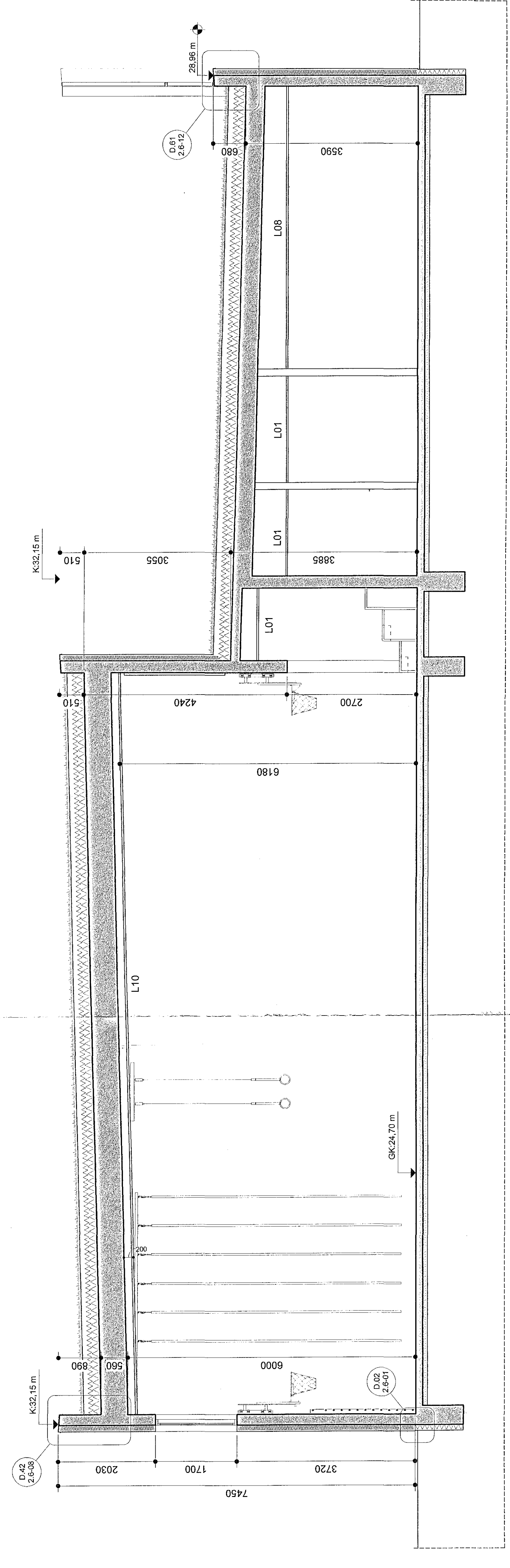
Sneiðing F1-F1 m.k.v. 1 : 50
