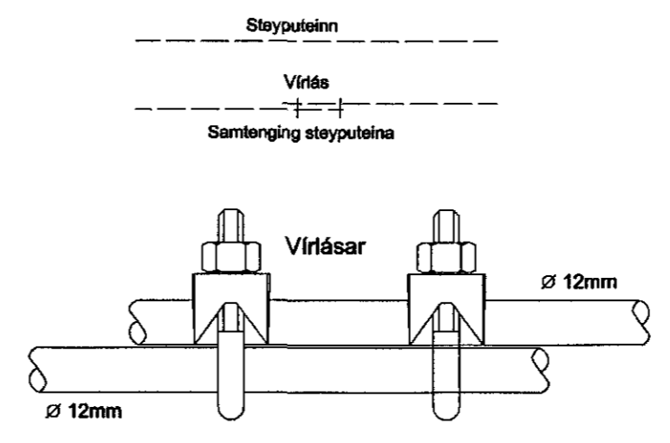
Samtenging steyptuina
