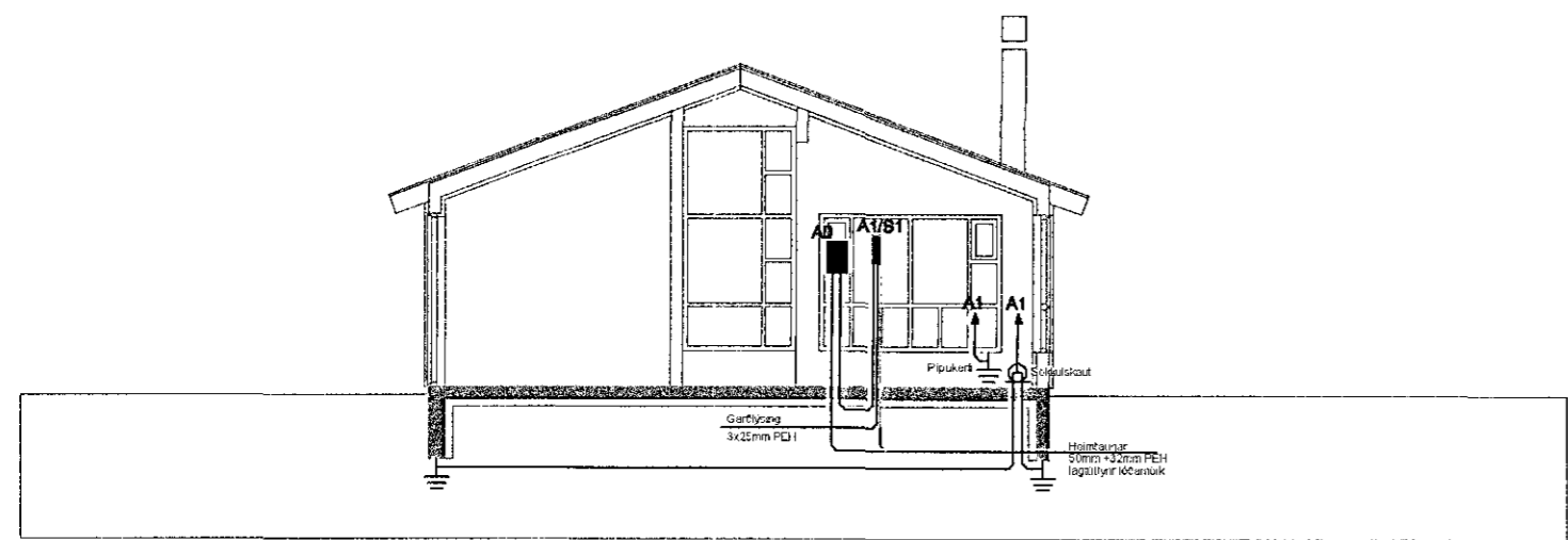
Sneiding A-A
