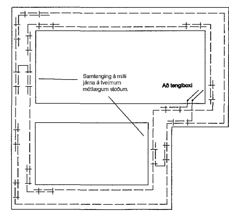
Grunnmynd sökkulveggja
