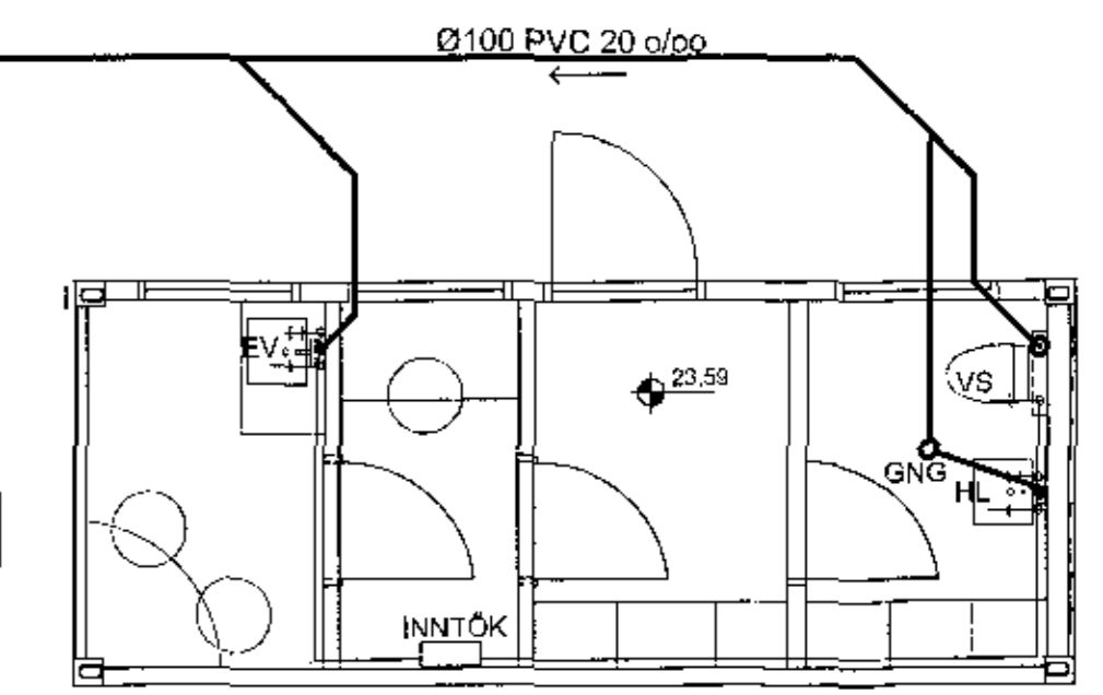
Starfsmannaaðstaða Mkv. 1:50
