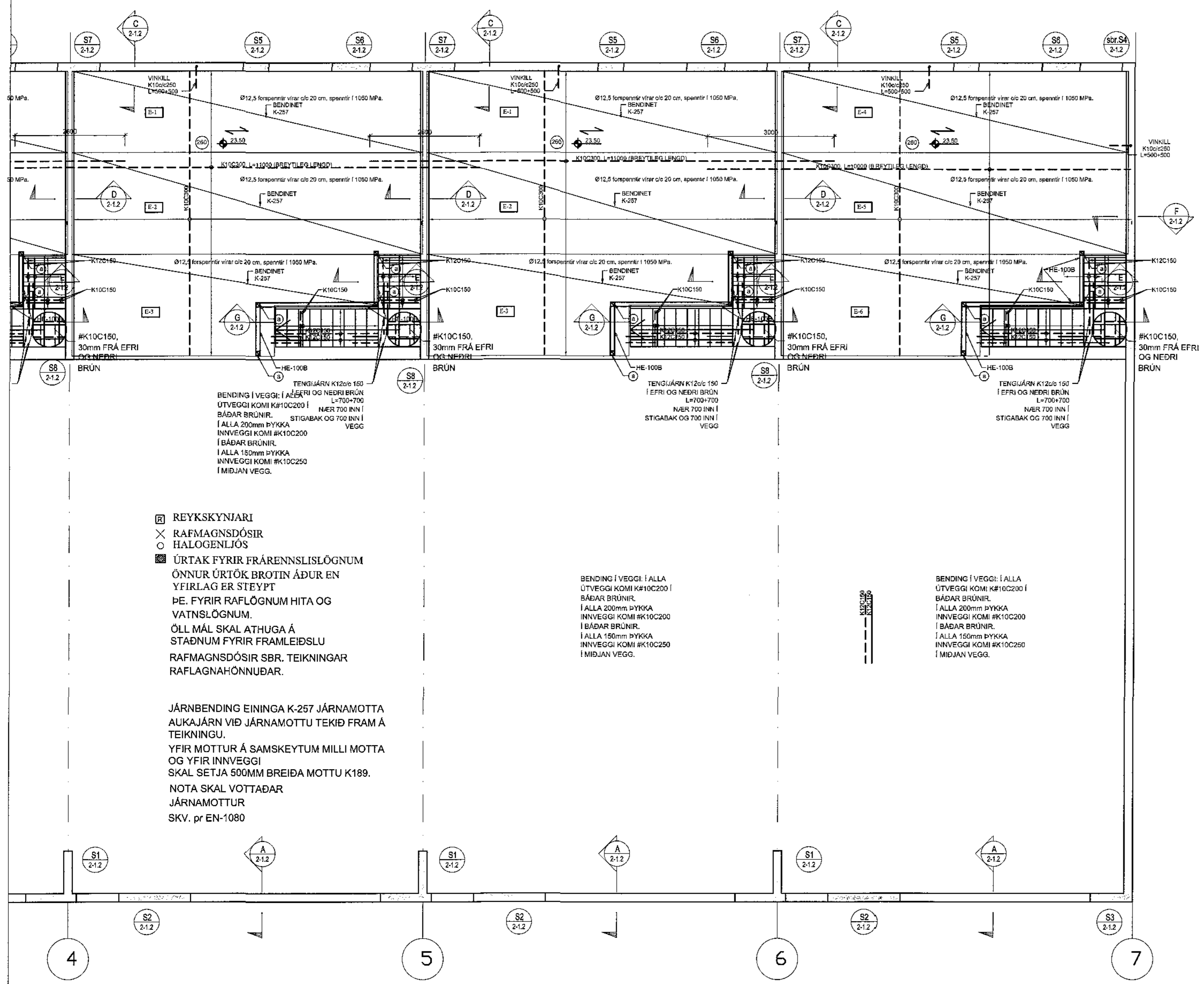
GRUNNMYND MILLIPLÖTU, 1:50
