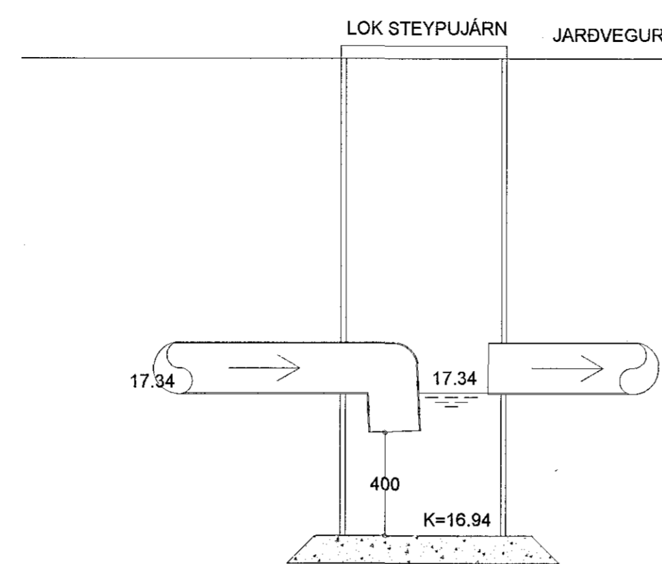
600mm VATNSLÁSABRUNNUR mkv. 1:20
