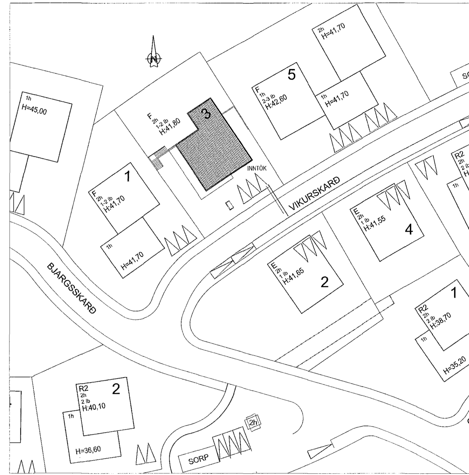
AFSTÖÐUMYND, MKV. 1:500
