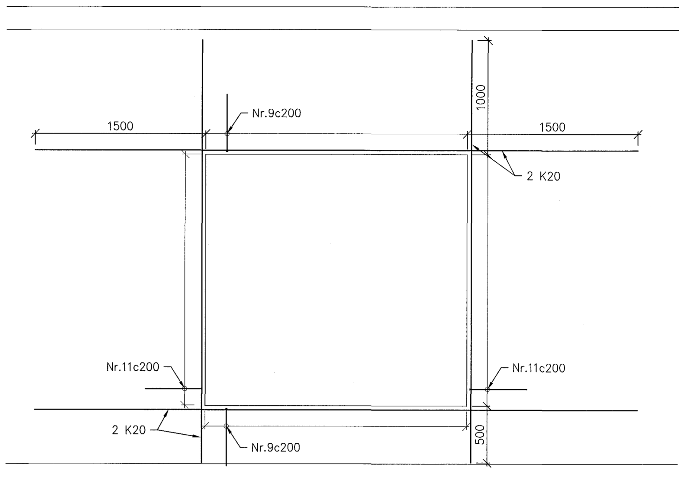
DEILI VIÐ HURÐAGÖT 2300x2200 1:20
