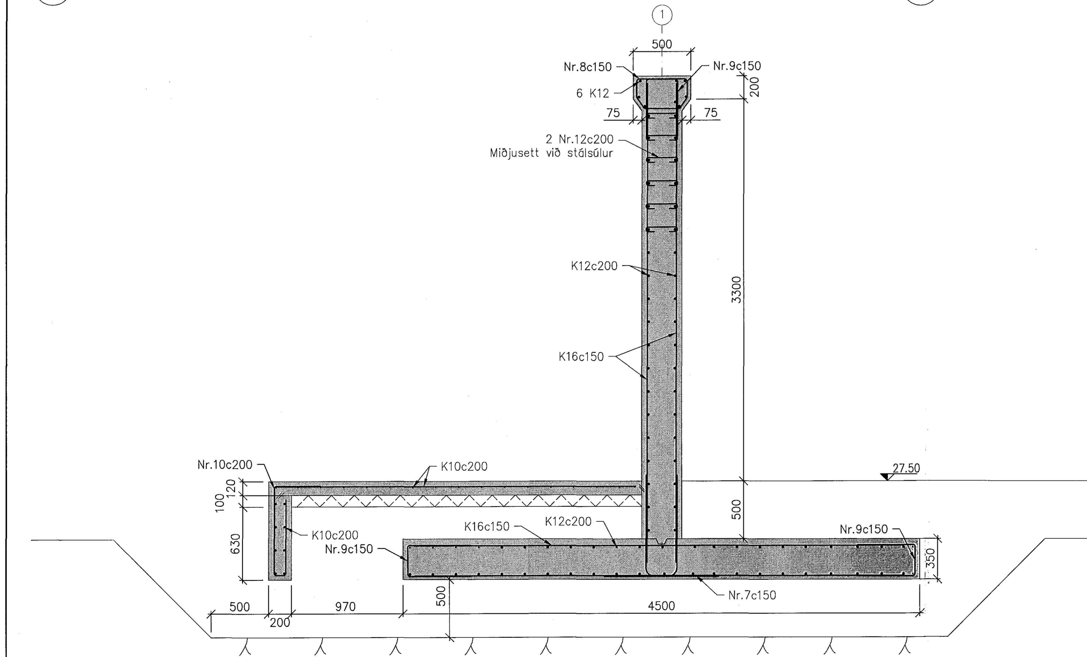
b SNID 101 1:20
