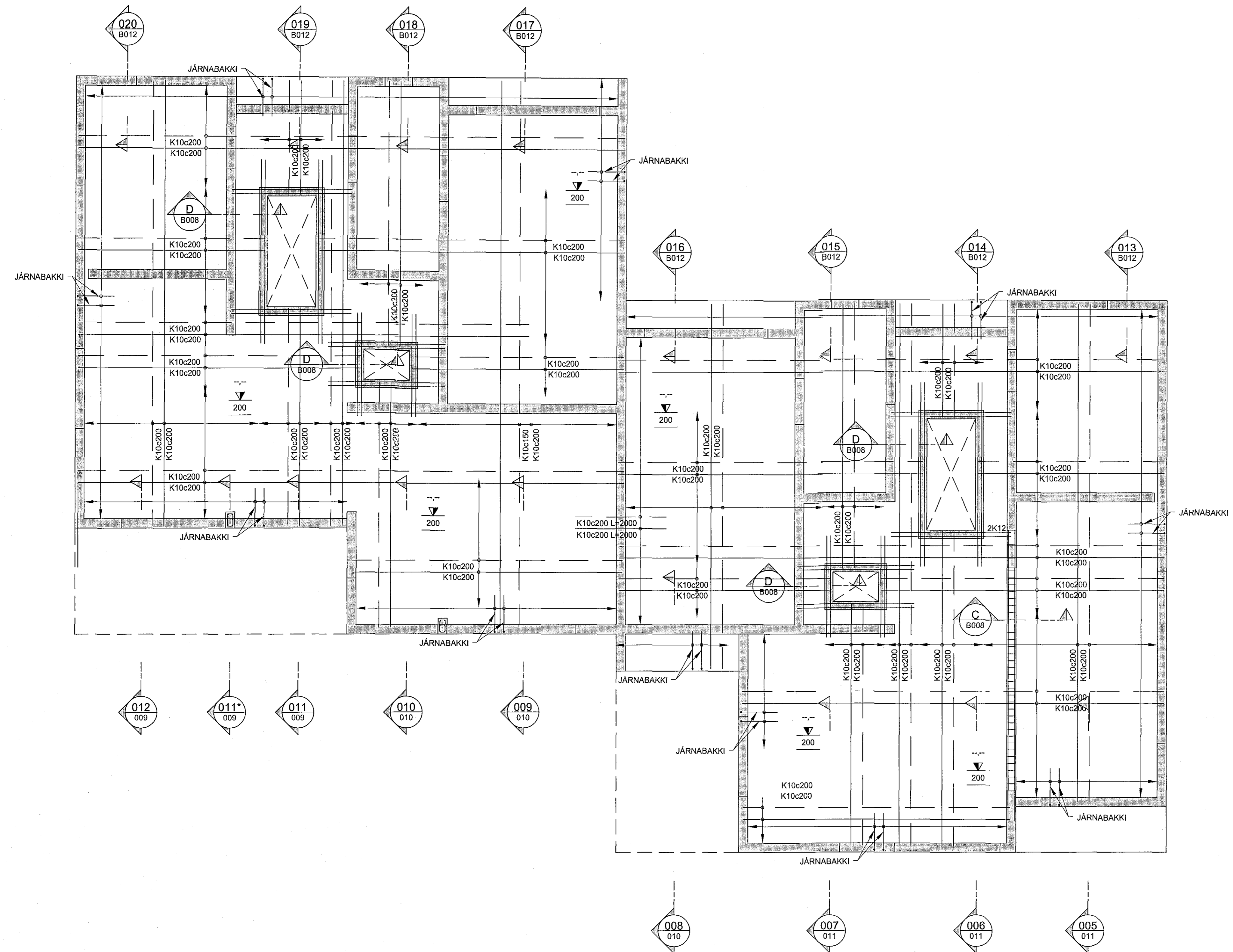
GRUNNMYND - STEINSTEYPT PLATA YFIR 2.HÆÐ 1:50 (A1)
