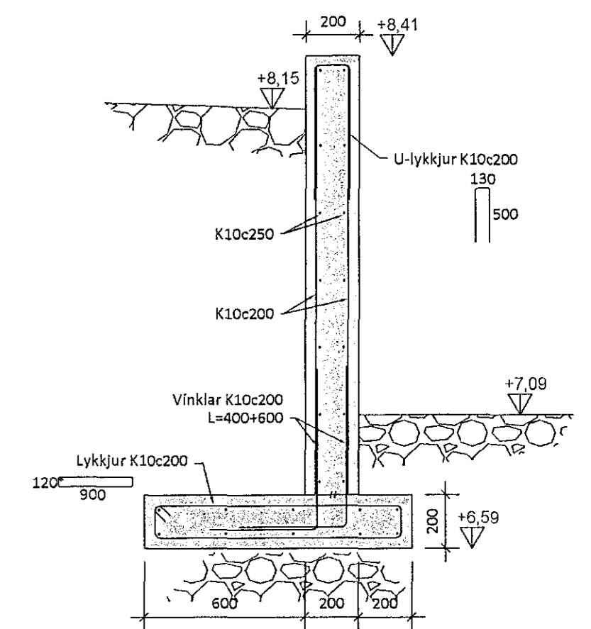
SNID Í STOVVEGG Mkv. 1:20
