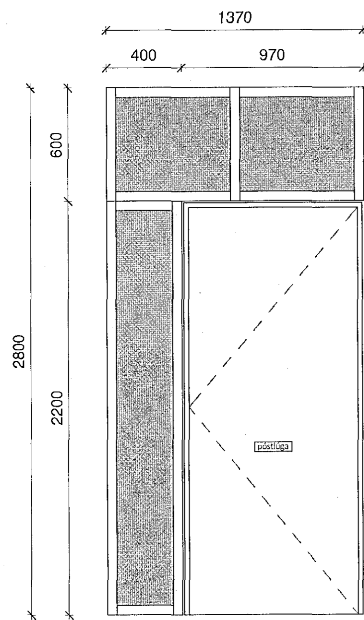
6 Útihurð stell - 2 stk 1 : 20
