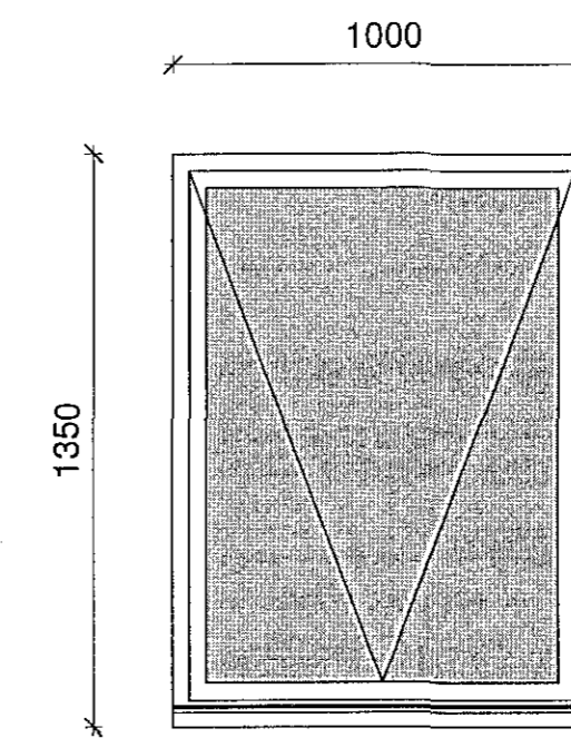
4 GL-4 - 6 stk - opnanlegt fag 1 : 20
