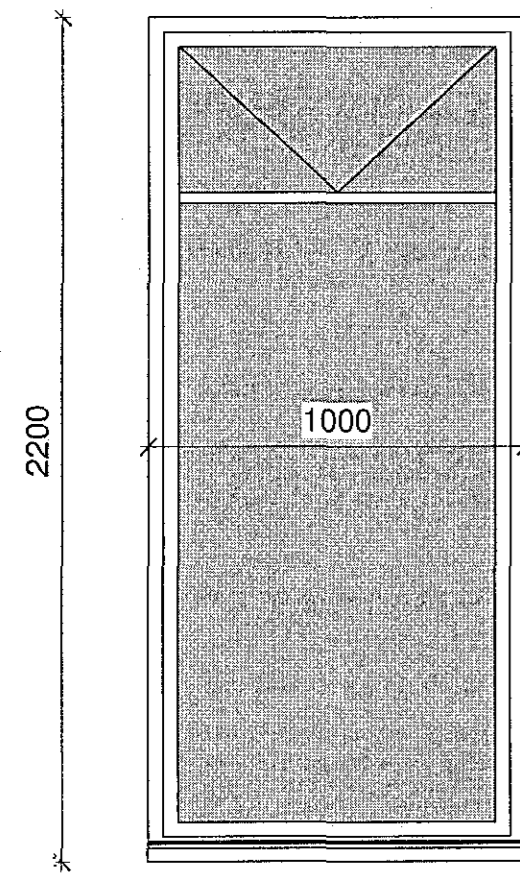
1 GL-1 - 2 stk - opnanlegt fag 1 : 20
