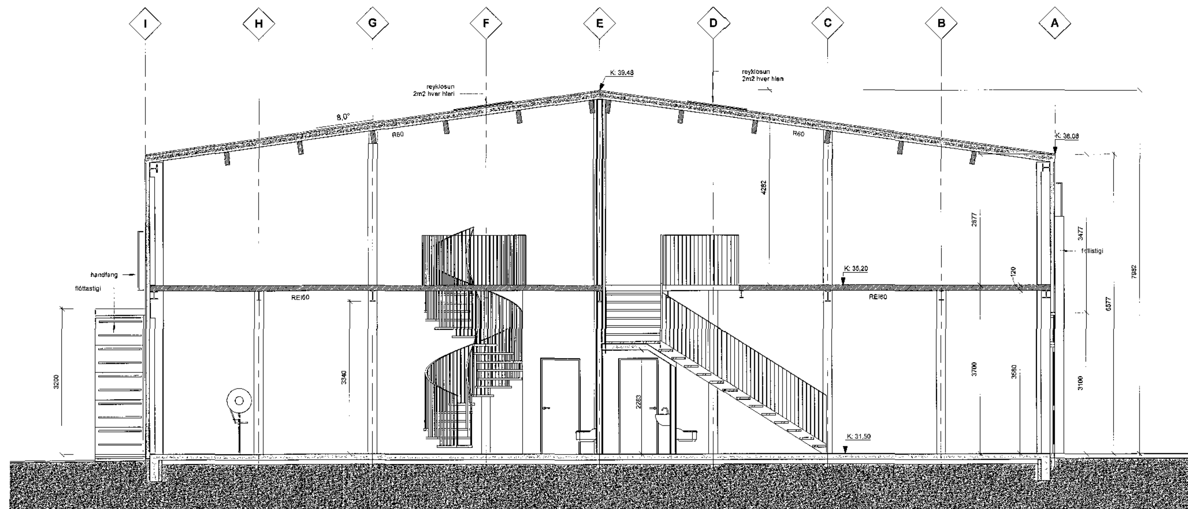
Snið AA_50 1:50
