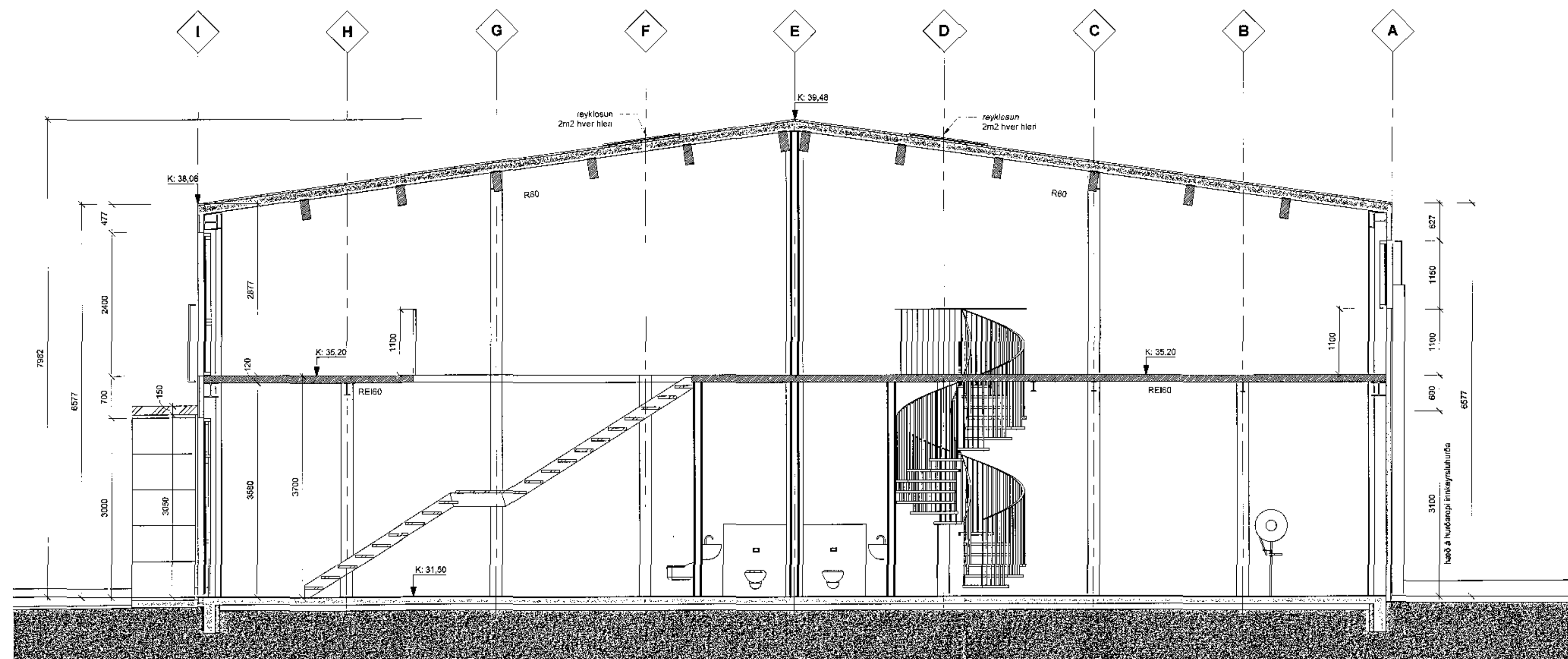
Snið BB_50 1:50
