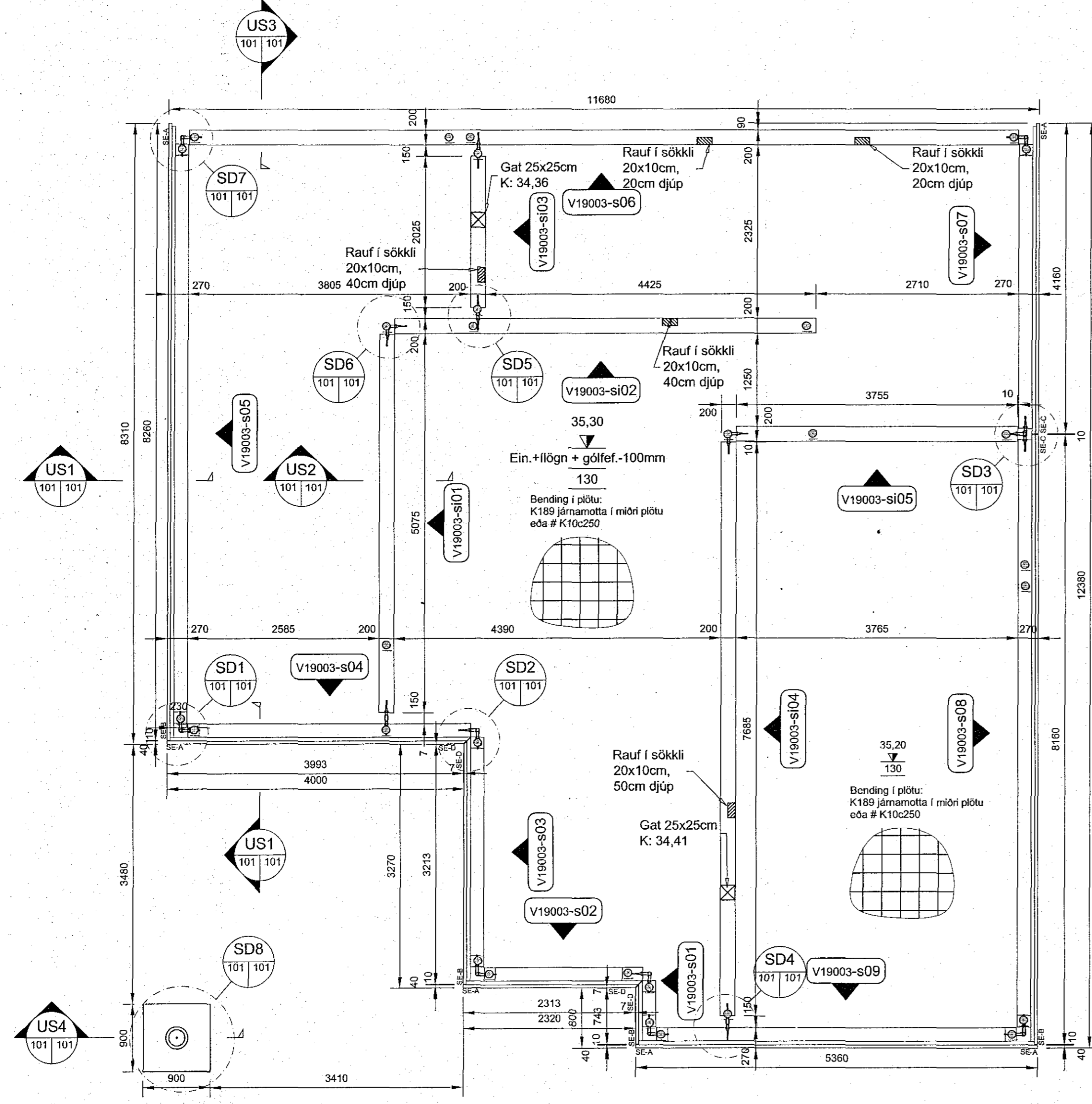
Grunnmynd sökklá 1:50
