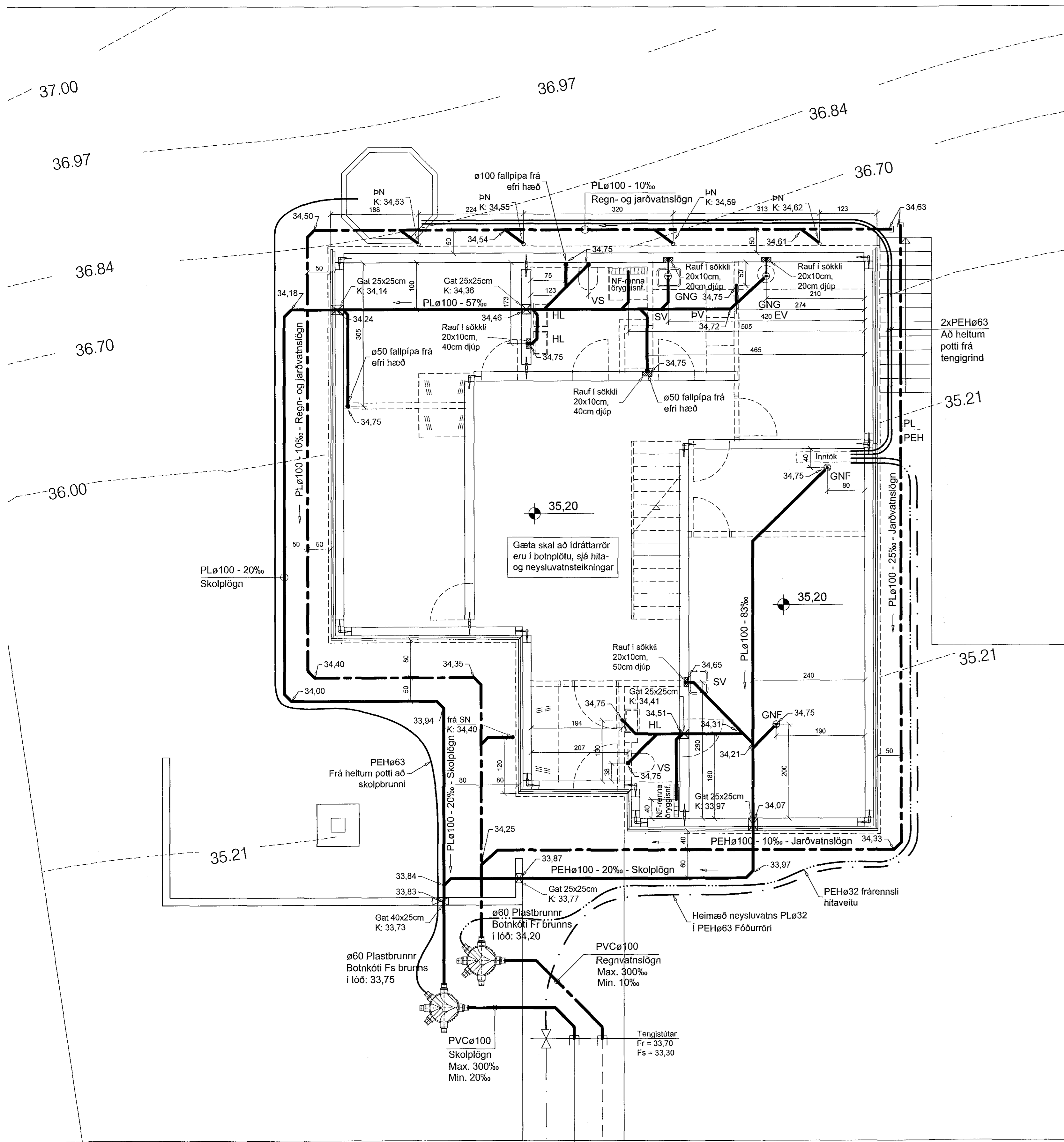
Afstöðumynd, mkv. 1:500
