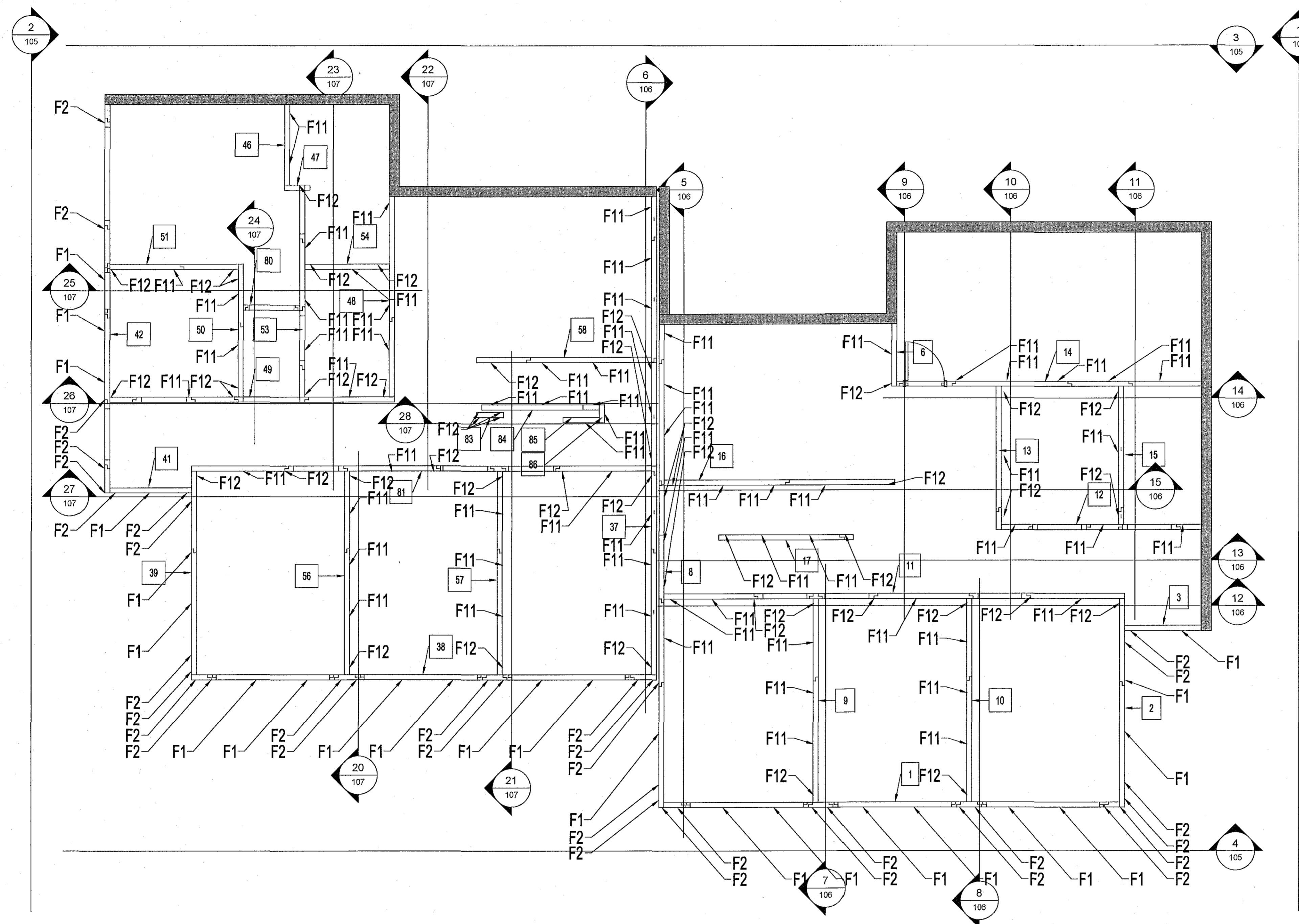
A PLAN - VEGGIR 1.HÆÐ 1:50
