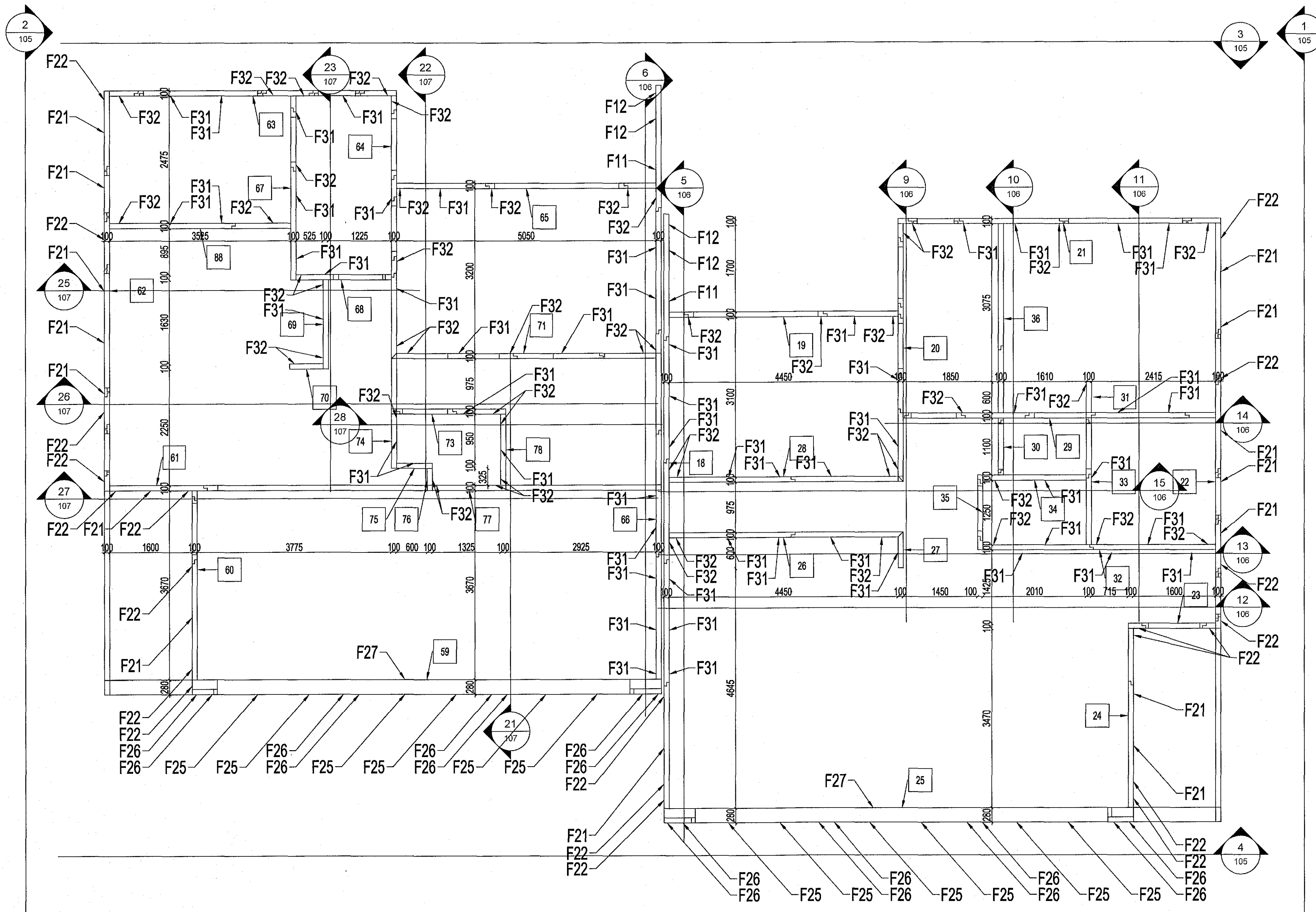
A PLAN - VEGGIR 2.HÆÐ 1:50
