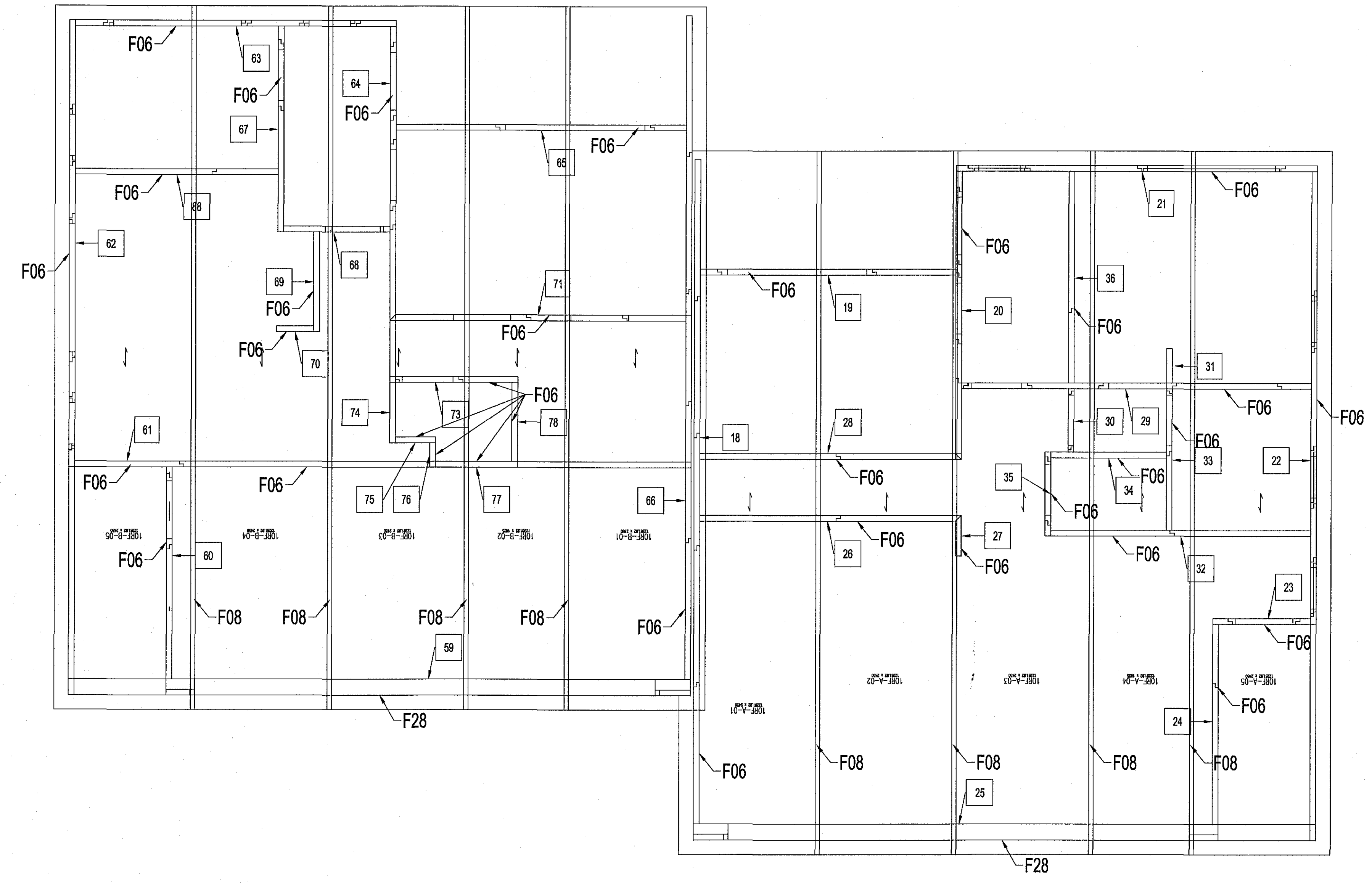
B PLAN - ÞAK 1:50
