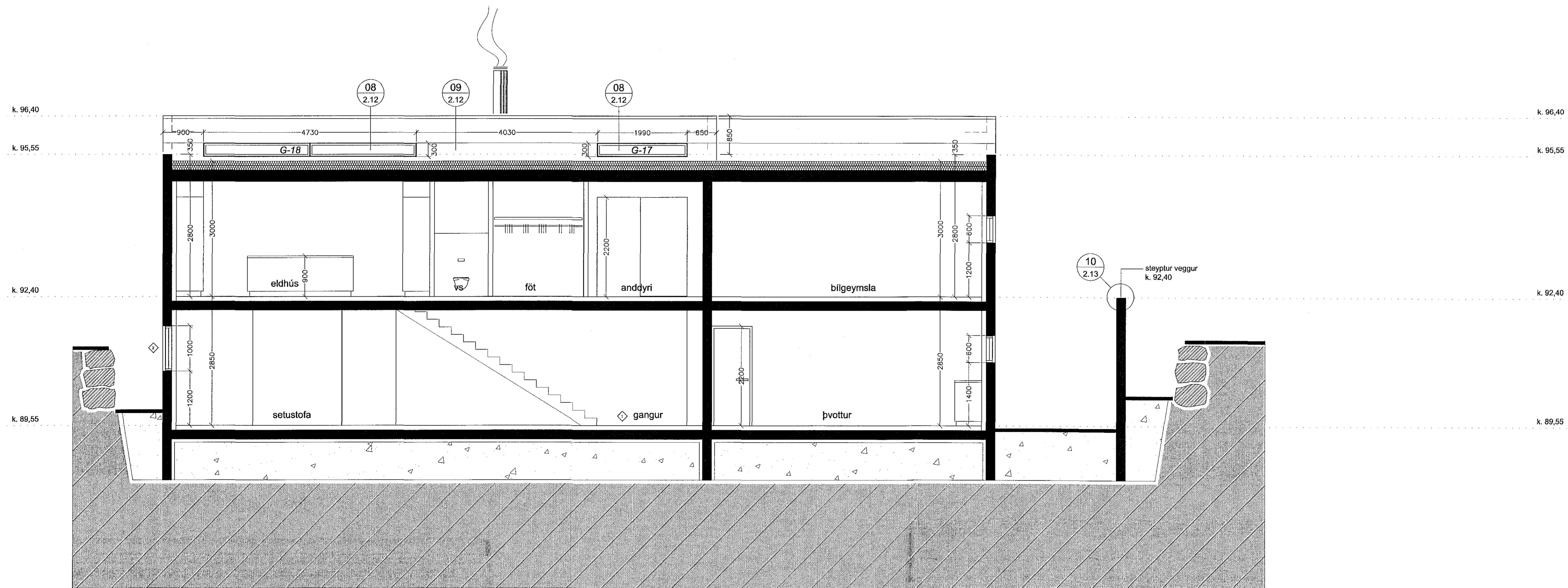
SNEIDING E - E M 1:50
