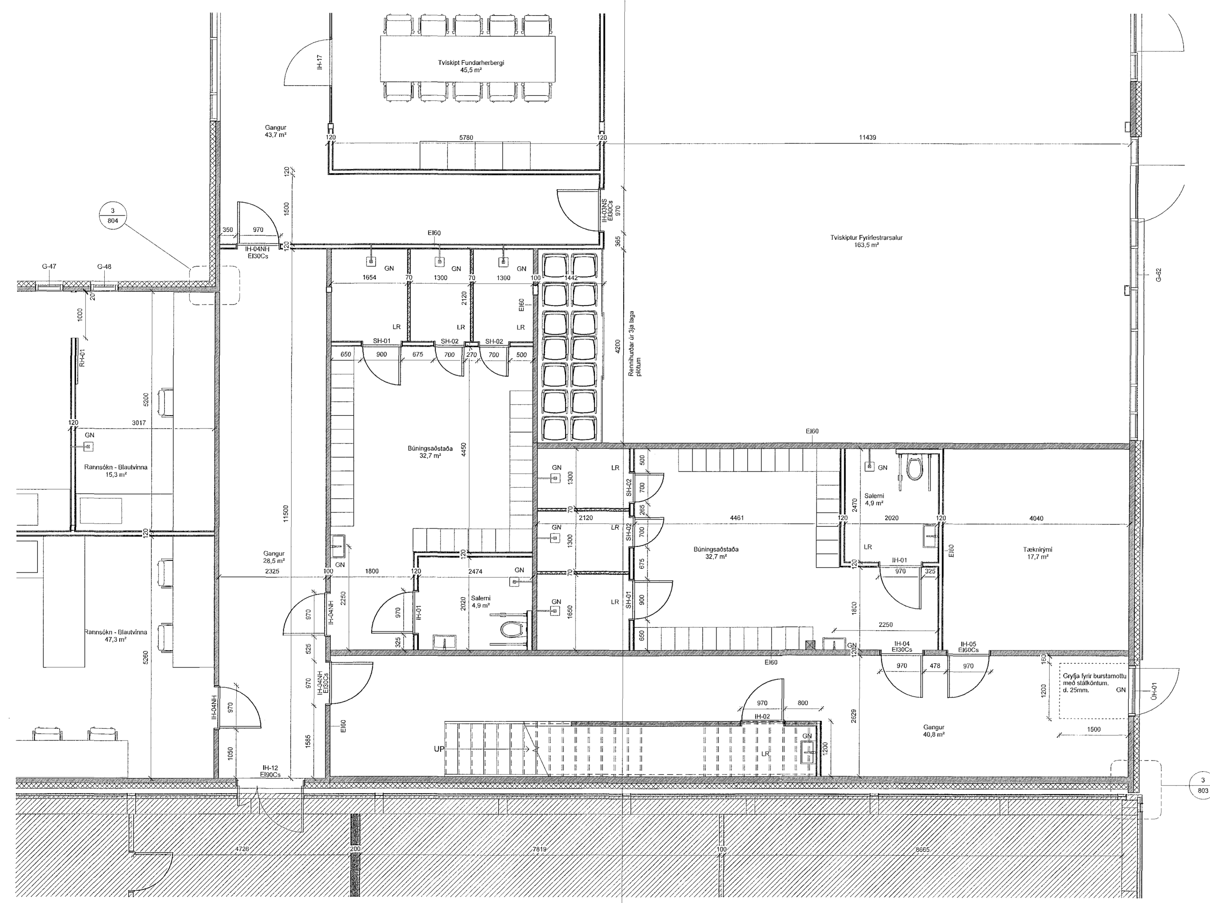
1 1.Hæð - Hluti C 1:50
