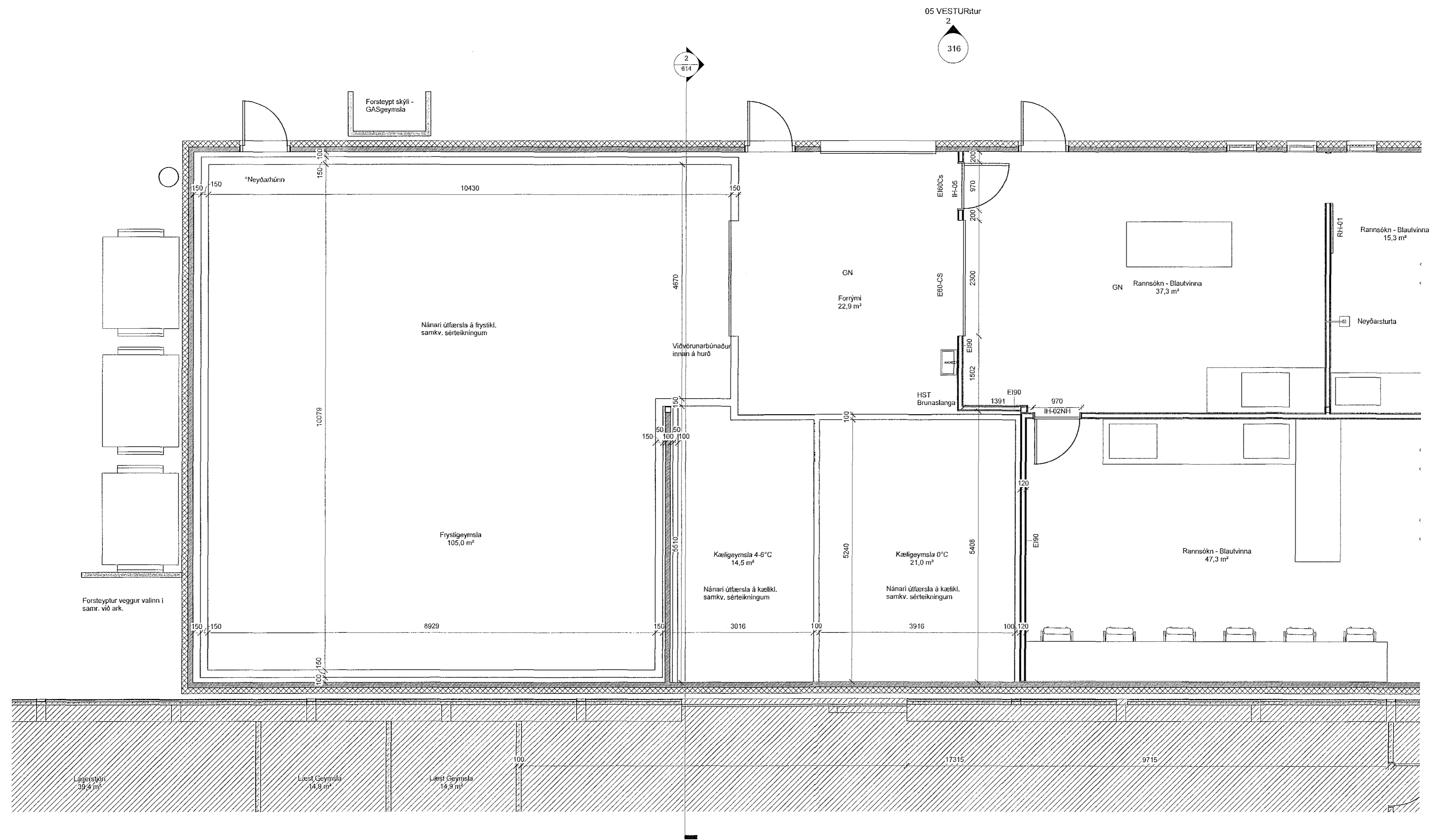
1 1.Hæð - Hluti D 1:50
