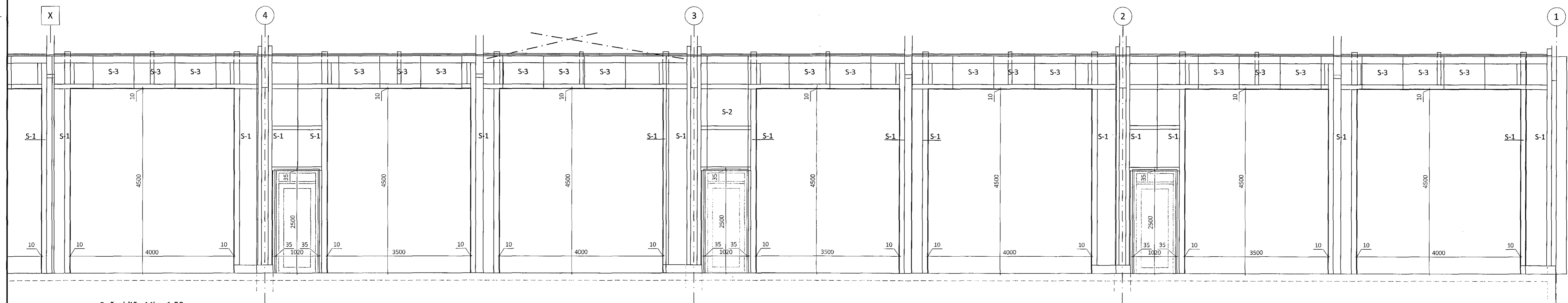
Suðurhlíð - Mkv. 1:50
