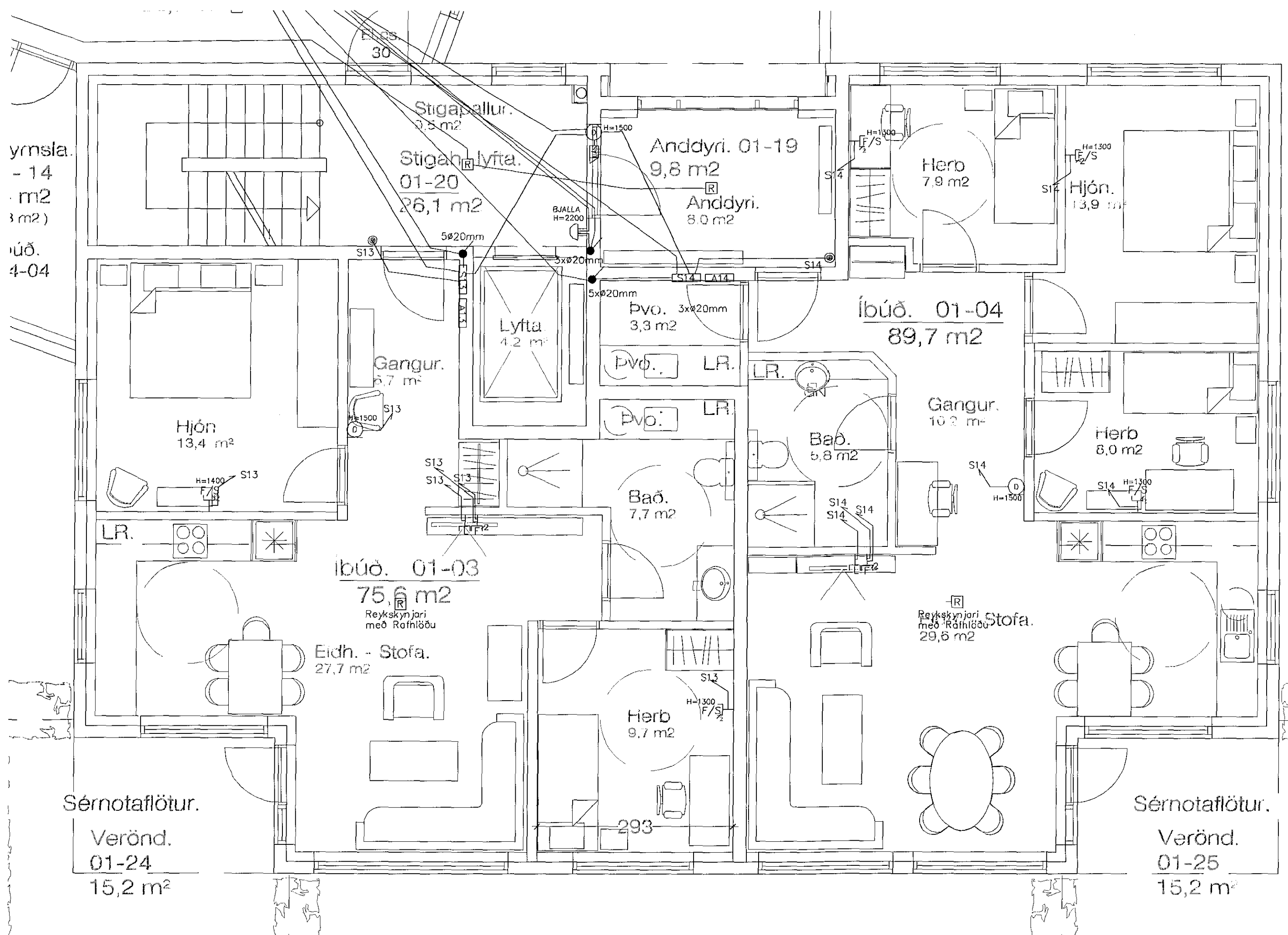
Grunnmynd íbúðir 103 og 104: 1:50
