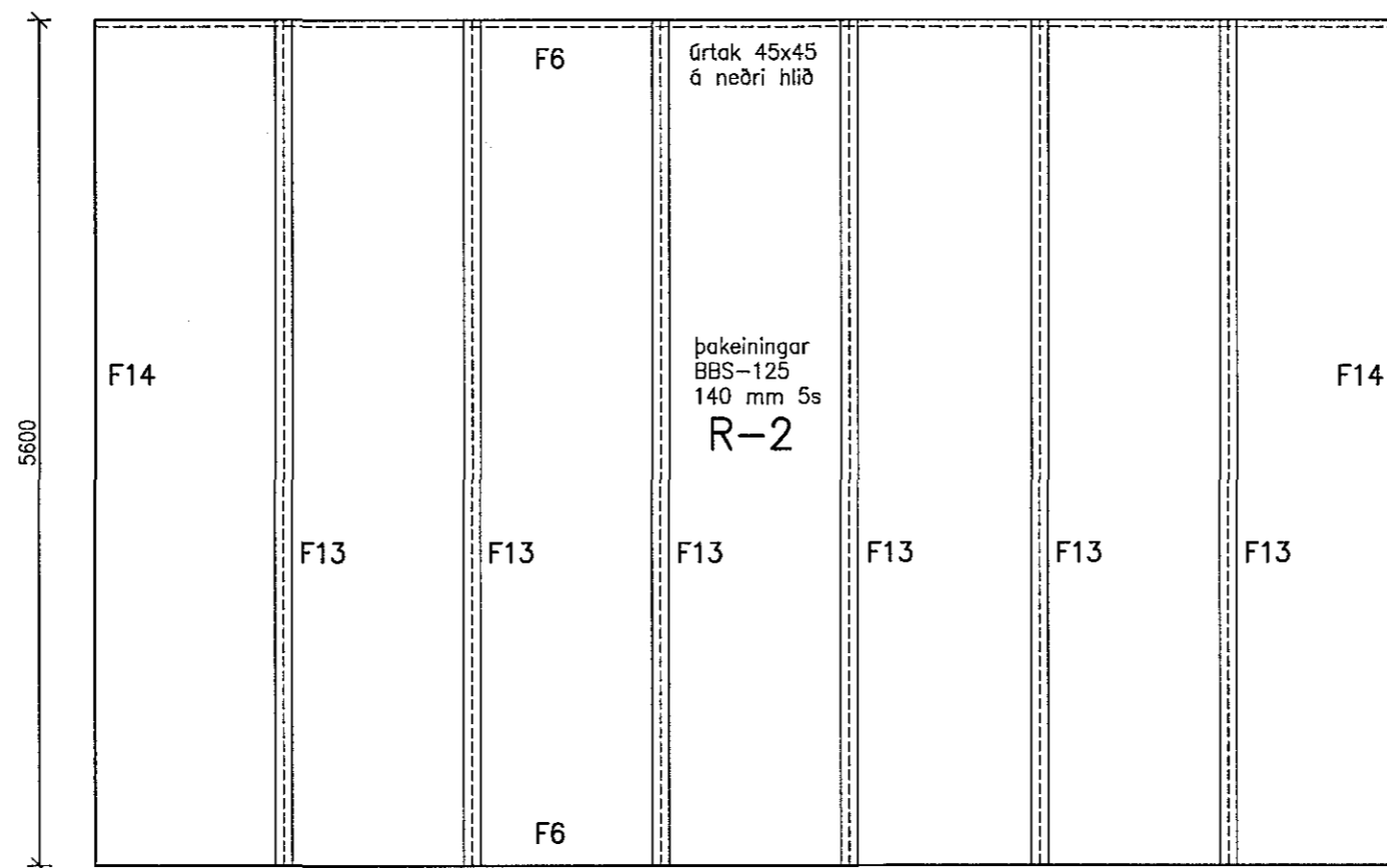
ÞAKEININGAR 1:50
