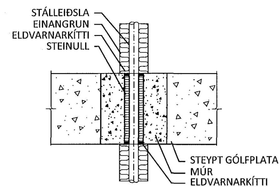
DÆMIGERÐ ÞÉTTING Á STÁLLÖGN Í GEGNUM STEYPT GÓLF (HÆÐARSKIL) (EKKI Í KVARÐA)
