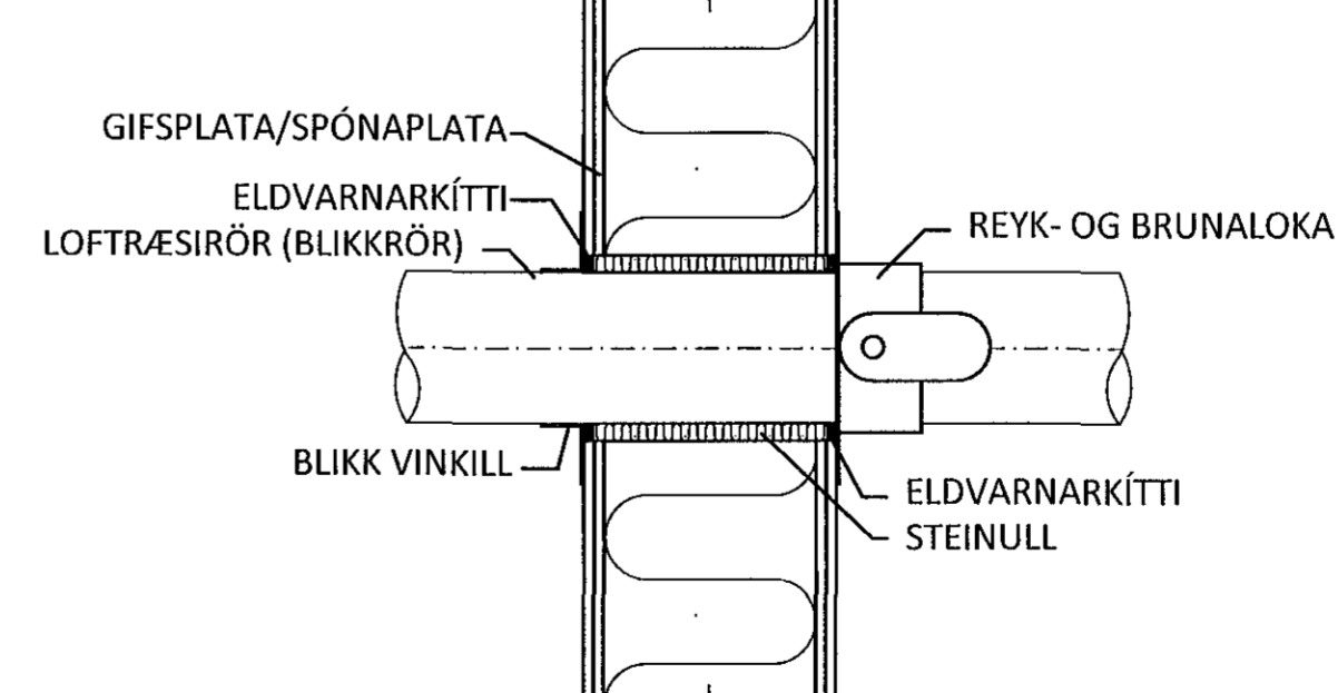
DÆMIGERÐ ÞÉTTING Á LOFTRÆSILÖGN Í GEGNUM LÉTTAN BRUNAVEGG (EKKI Í KVARÐA)
