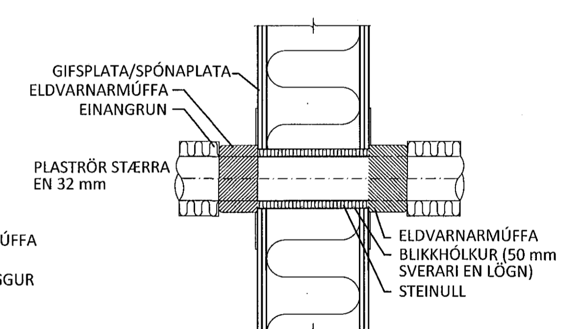
DÆMIGERÐ ÞÉTTING Á PLASTLÖGN STÆRRI EN 32 mm Í GEGNUM LÉTTAN BRUNAVEGG (EKKI Í KVARÐA)
