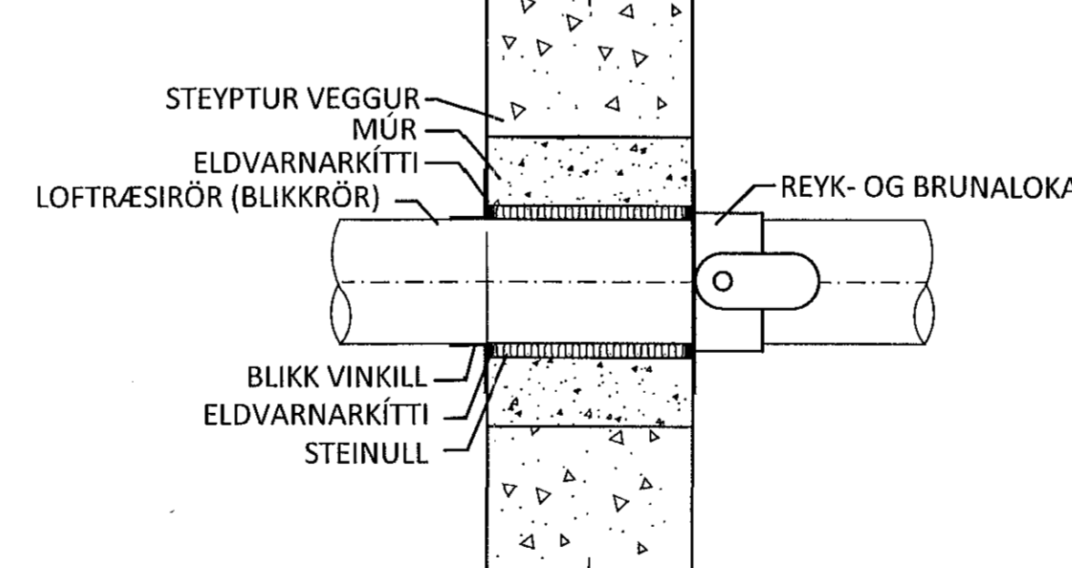
DÆMIGERÐ ÞÉTTING Á LOFTRÆSILÖGN Í GEGNUM STEYPTAN BRUNAVEGG (EKKI Í KVARÐA)
