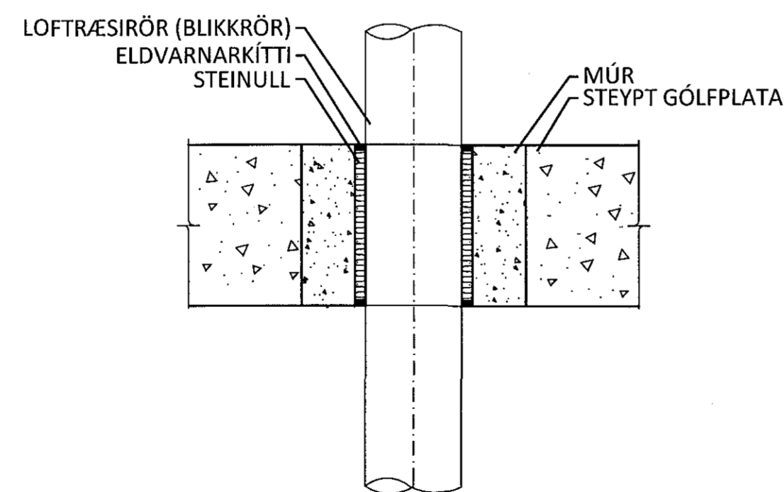
DÆMIGERÐ ÞÉTTING Á LOFTRÆSILÖGN Í LAGNASKAKTI Í GEGNUM STEYPTAN BRUNAVEGG (EKKI Í KVARÐA)
