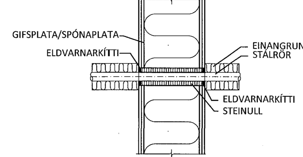
DÆMIGERÐ ÞÉTTING Á STÁLLÖGN Í GEGNUM LÉTTAN BRUNAVEGG (EKKI Í KVARÐA)
