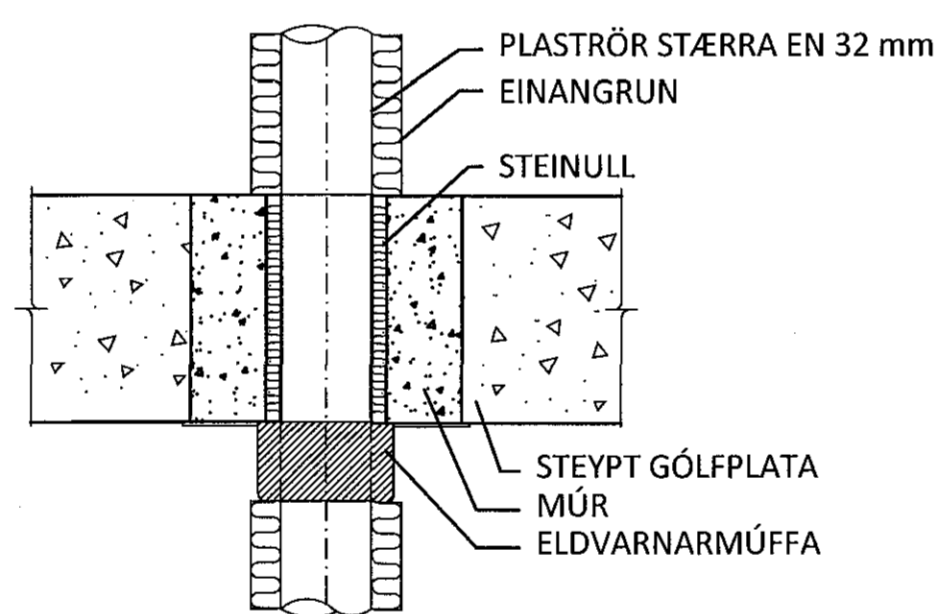
DÆMIGERÐ ÞÉTTING Á PLASTLÖGN STÆRRI EN 32 mm Í GEGNUM STEYPT GÓLF (HÆÐARSKIL) (EKKI Í KVARÐA)
